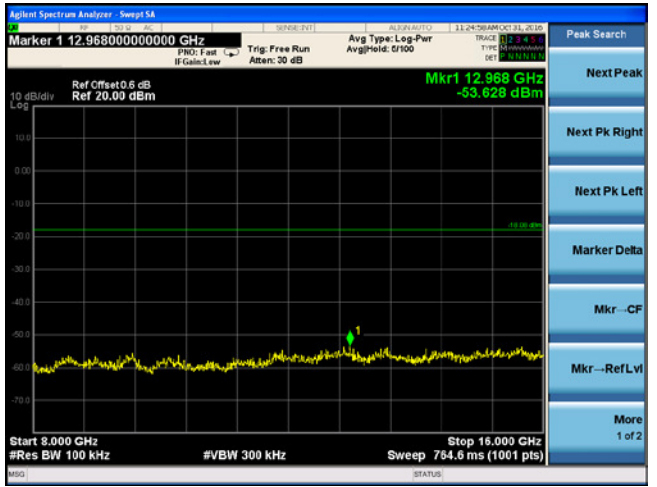
8GHz~16GHz
