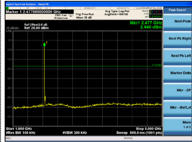
1GHz~8GHz
