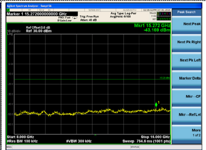
8GHz~16GHz
