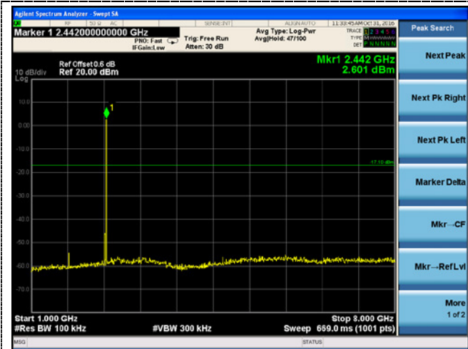
1GHz~8GHz
