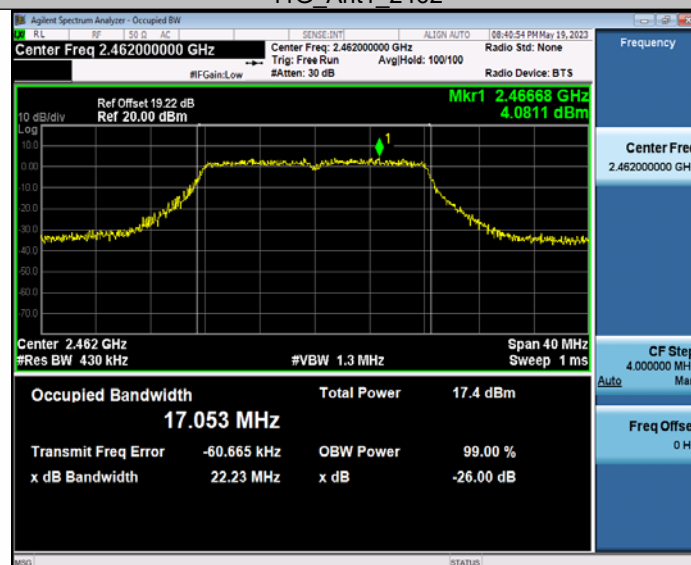
11G_Ant1_2462
