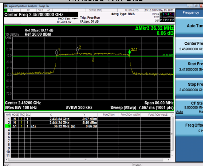
11N40SISO Ant1 2452
