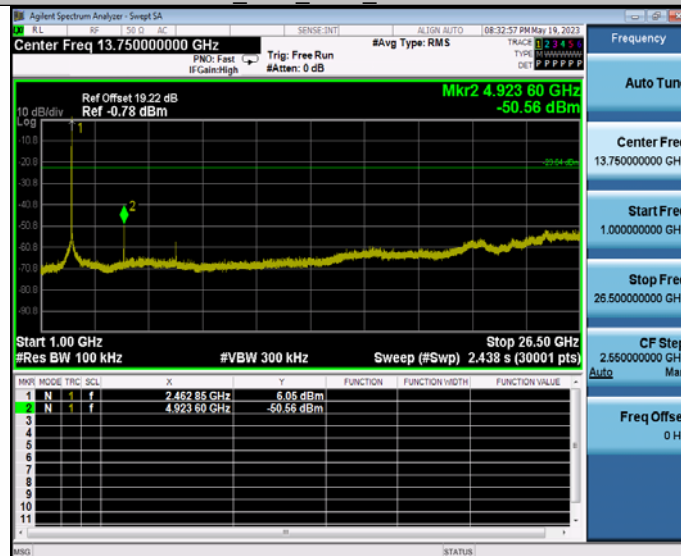
11B_Ant1_2462_1000~26500
