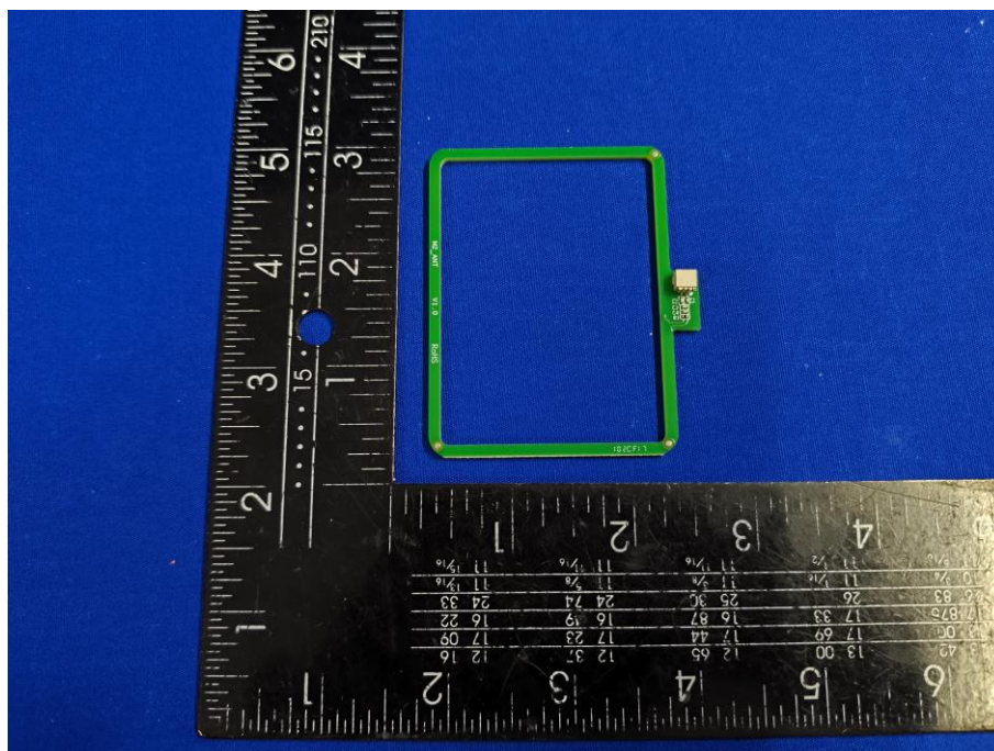
13.56M antenna
