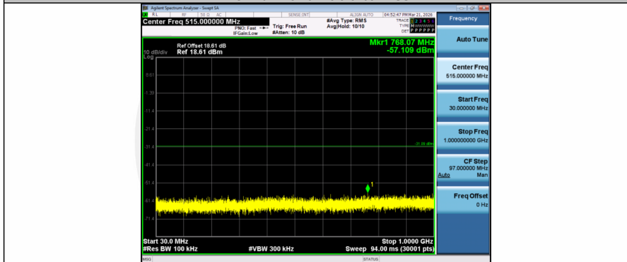
11G-Ant1-2437-30~1000-PASS
