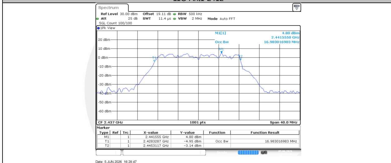
11G-Ant1-2437
