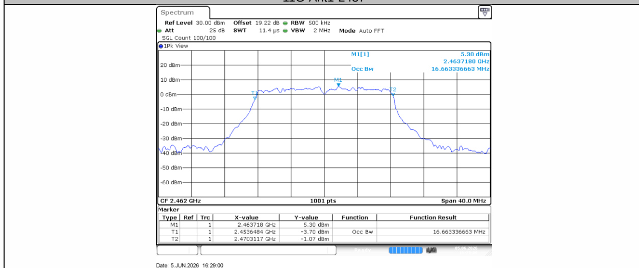
11G-Ant1-2462
