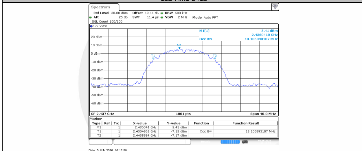
11B-Ant1-2437
