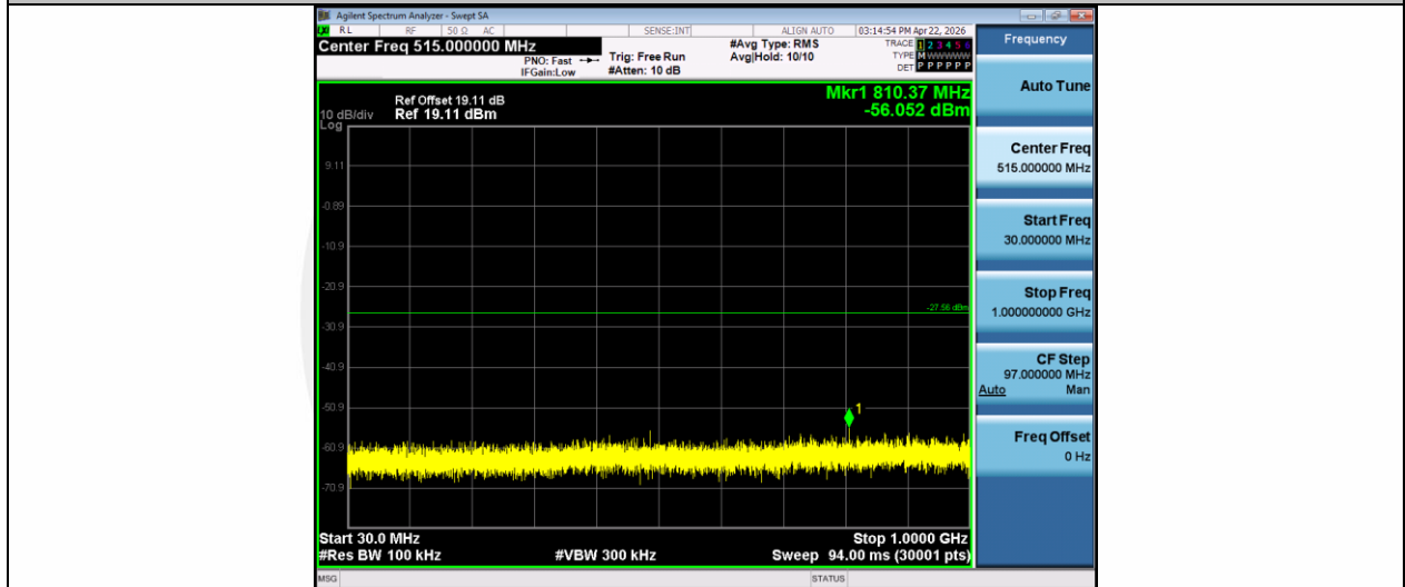
11G-Ant1-2437-30~1000-PASS
