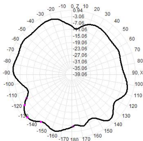
2400MHz
