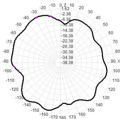
2500MHz
