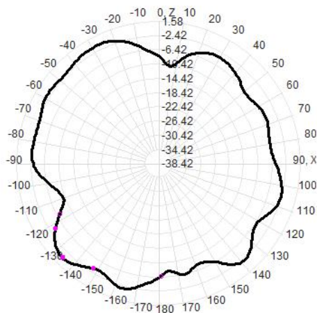
2450MHz
