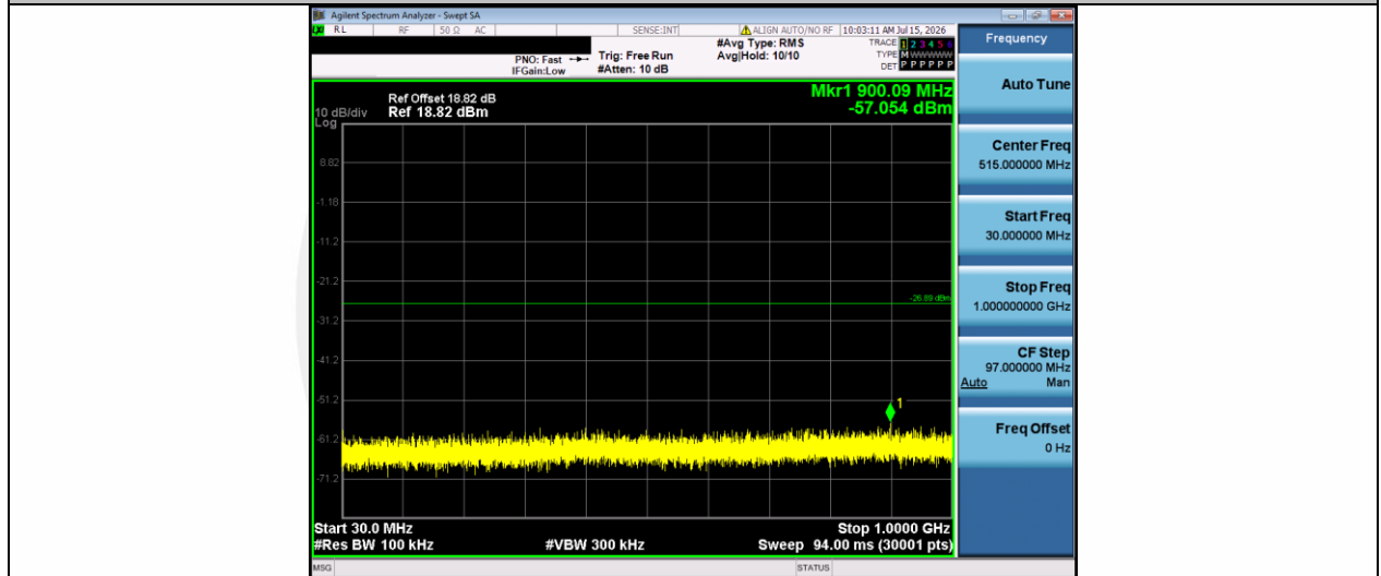
11G-Ant1-2462-30~1000-PASS
