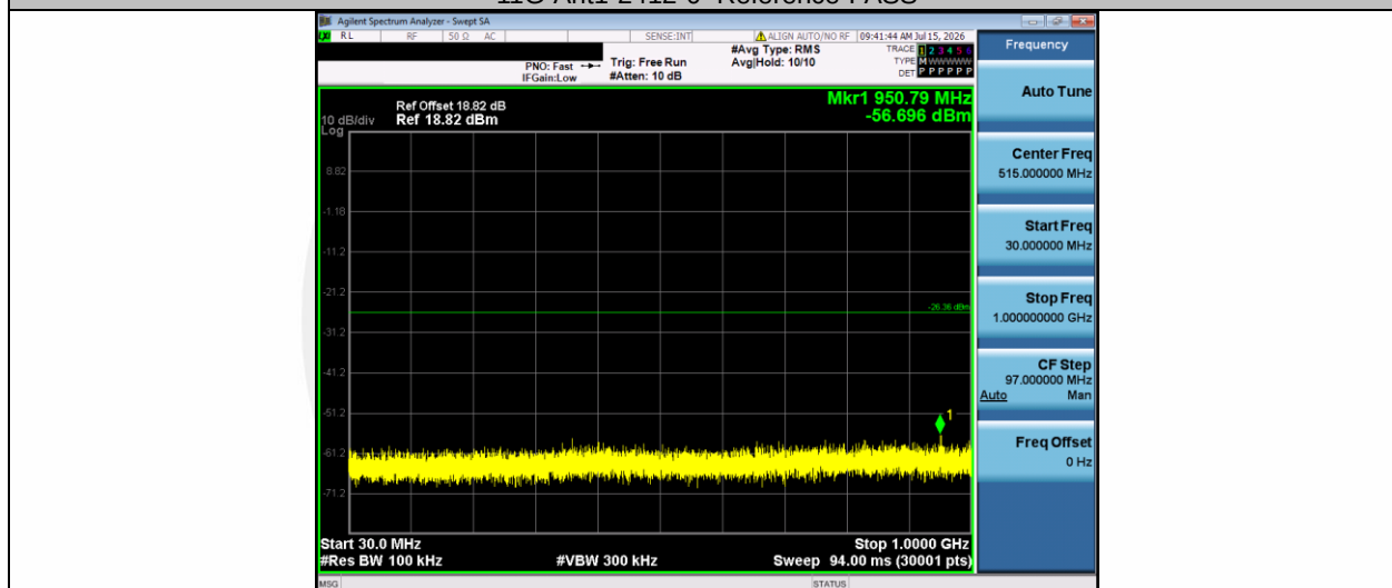
11G-Ant1-2412-30~1000-PASS
