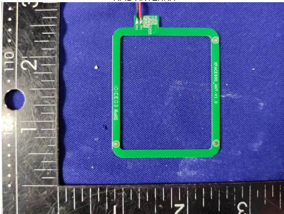
RFID ANTENNA
