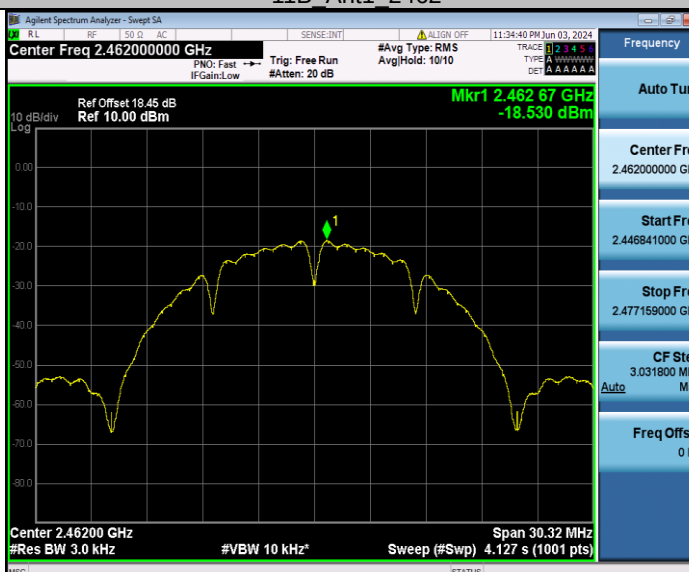
11B_Ant1_2462
