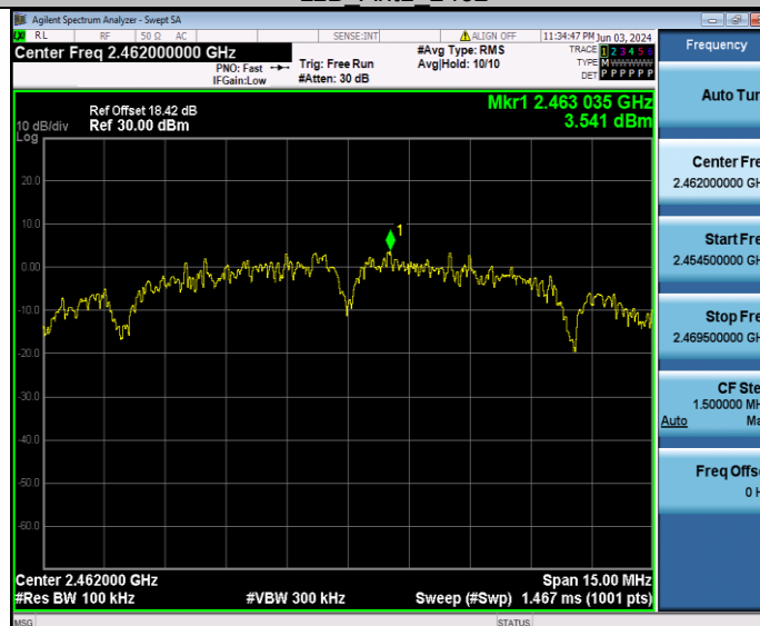
11B_Ant1_2462
