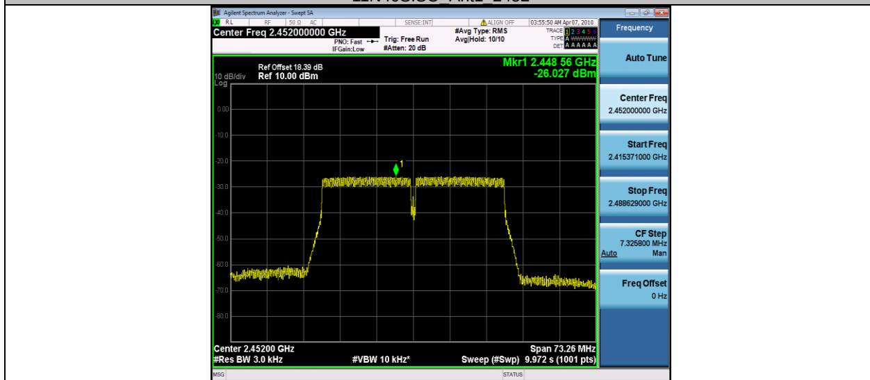
11N40SISO Ant1 2452
