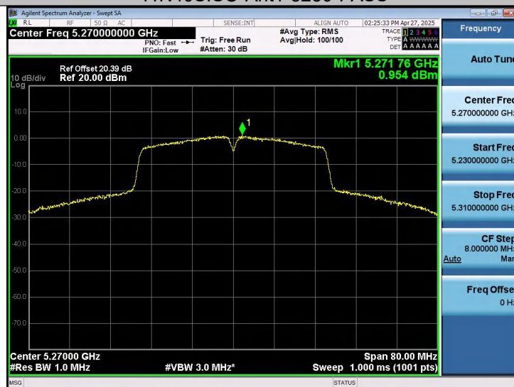
11N40SISO-Ant1-5270-PASS
