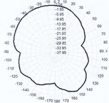
2400.0MHz Total(E1-XZ), Max=2.05dBi
