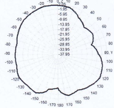
2400.0MHz Total(E2-YZ), Max=1.72dBi
