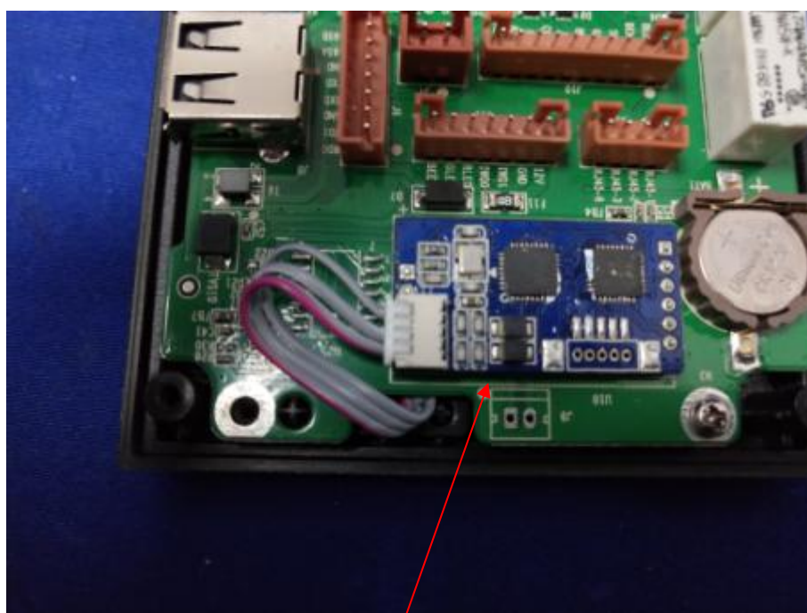
125KHz Module
