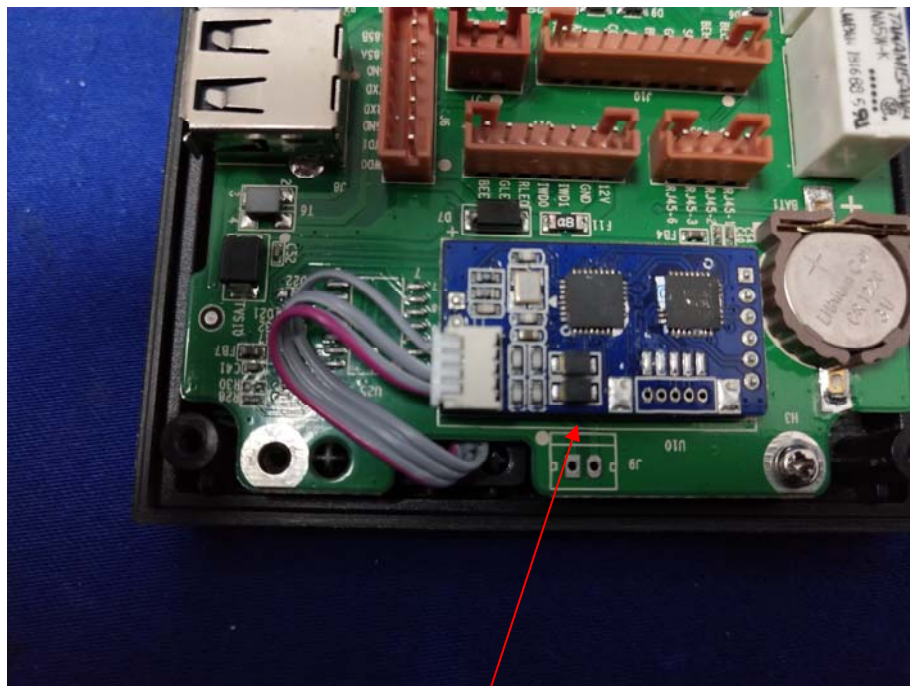
13.56MHz Module
