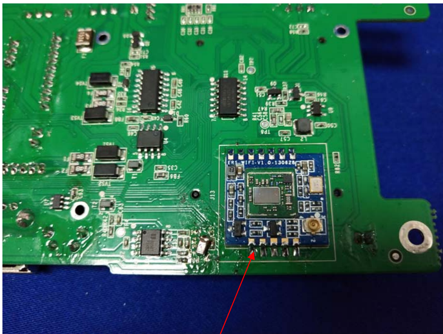
WIFI Module
