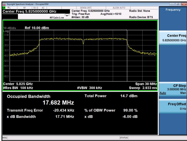
802.11 n(HT20) mode-ch165
