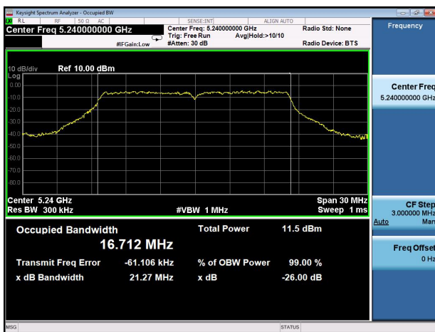
802.11a mode-ch48
