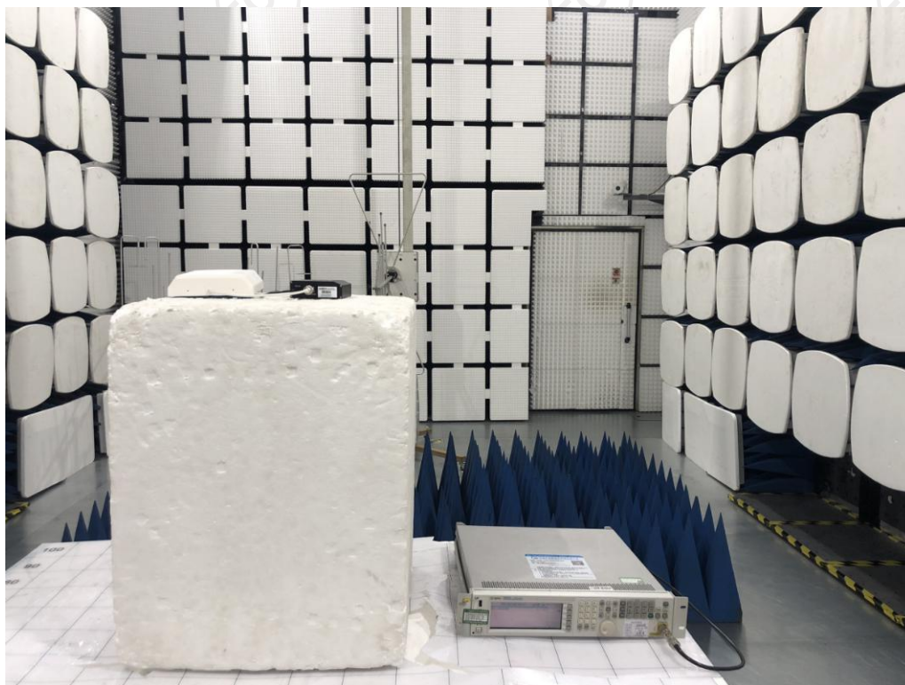
Fig. 2 (Below 1GHz)-SYN-OPA-8D
