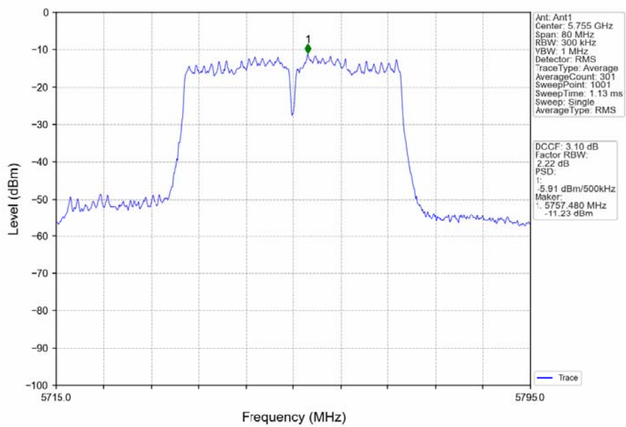
802.11ac(VHT40)_LCH_5755MHz_Ant1_NTNV
