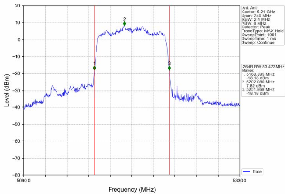
802.11ac(VHT80)_MCH_5210MHz_Ant1_NTNV
