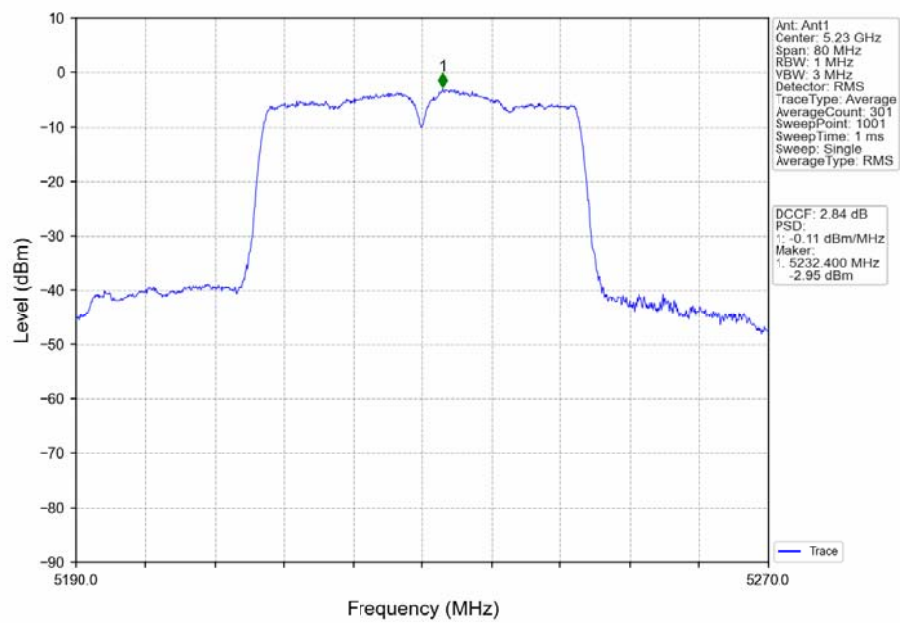
802.11n(HT40)_HCH_5230MHz_Ant1_NTNV
