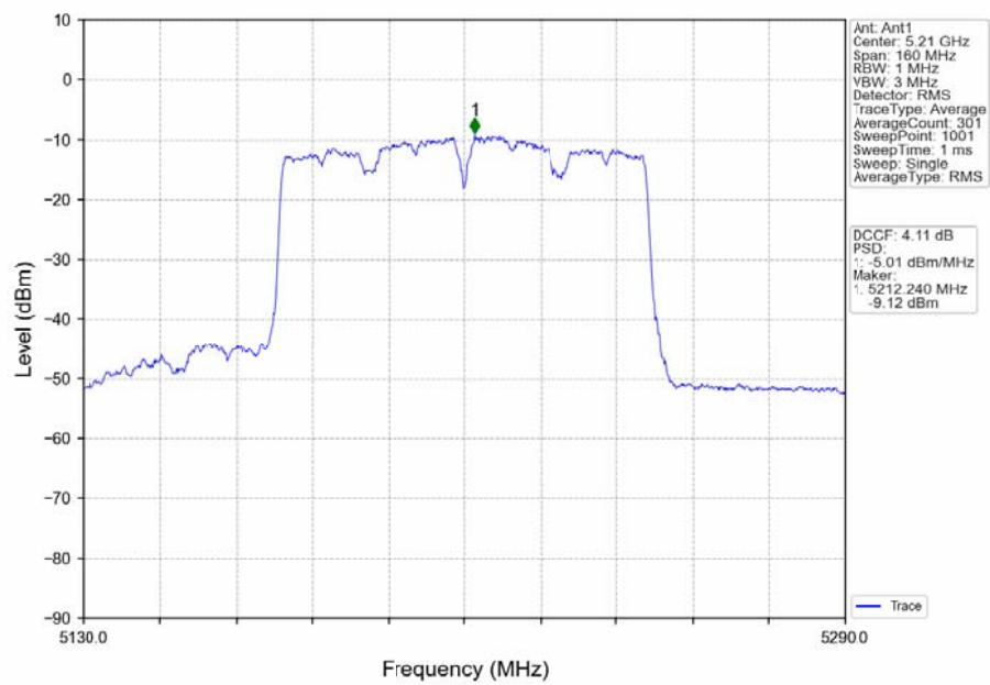
802.11ac(VHT80)_MCH_5210MHz_Ant1_NTNV
