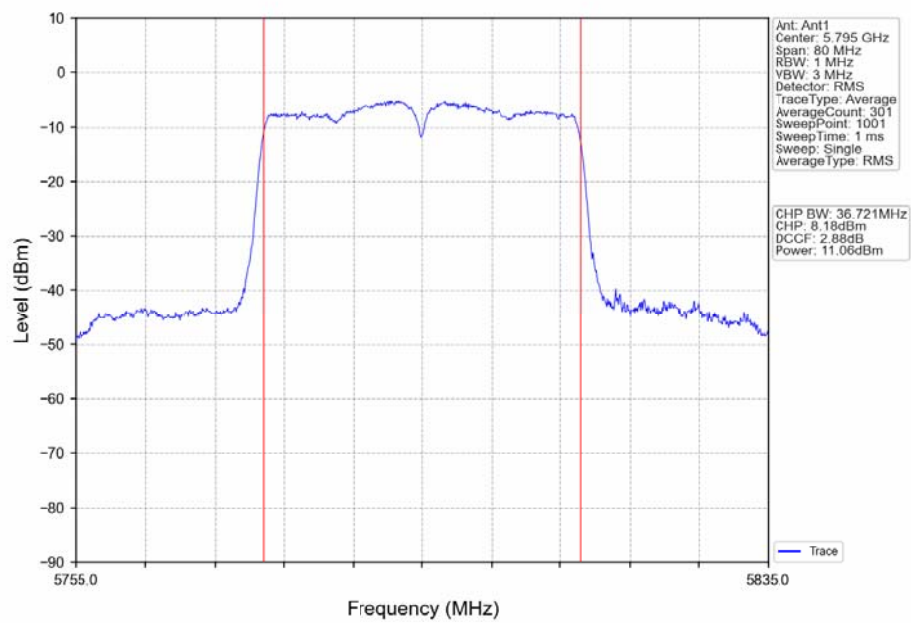
802.11n(HT40)_HCH_5795MHz_Ant1_NTNV
