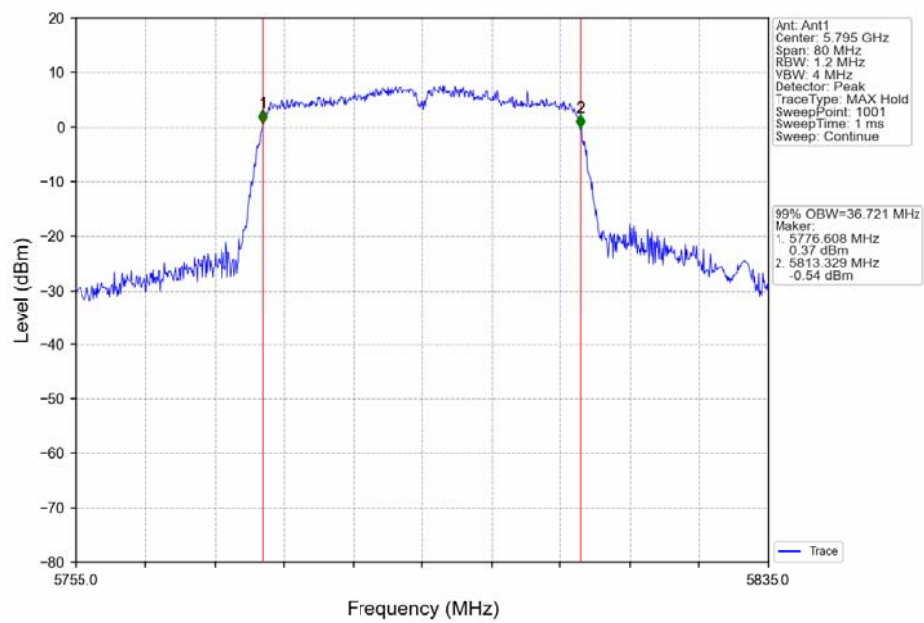
802.11n(HT40)_HCH_5795MHz_Ant1_NTNV
