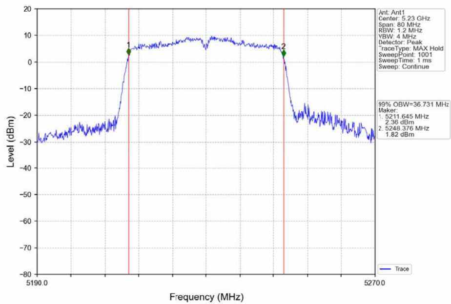
802.11n(HT40)_HCH_5230MHz_Ant1_NTNV
