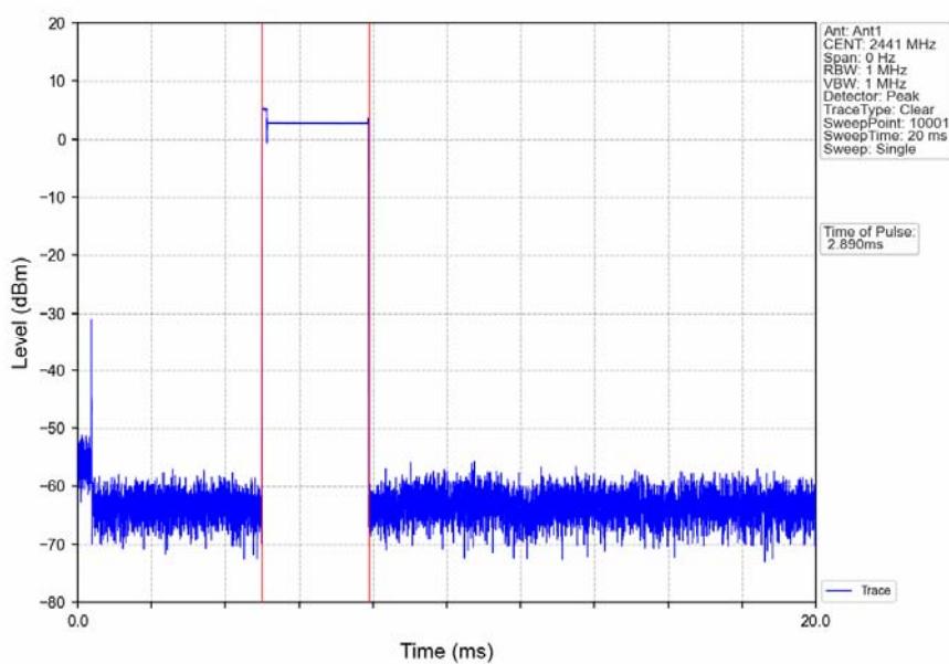
\pi/4 -DQPSK 2DH5 2441MHz
