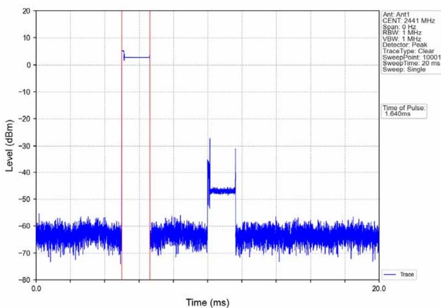
\pi/4 -DQPSK 2DH3 2441MHz
