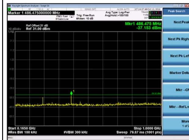
AIS2 165MHz - 1GHz
