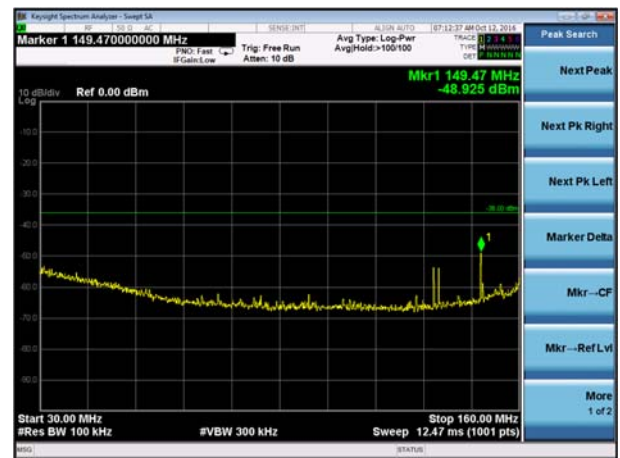
AIS2 30MHz - 160MHz
