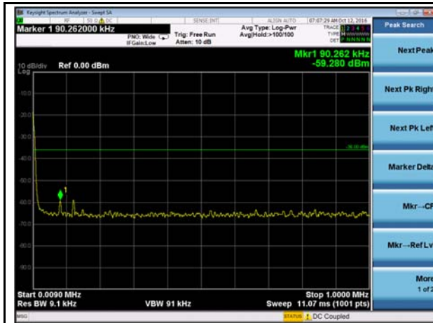
AIS1 9KHz - 1MHz
