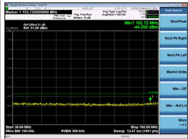
AIS1 30MHz - 160MHz
