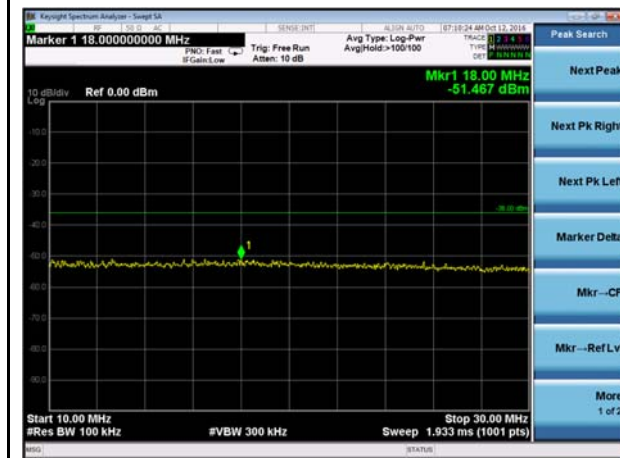
AIS2 10MHz - 30MHz
