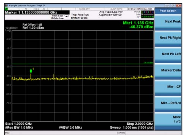
AIS2 1GHz - 2GHz
