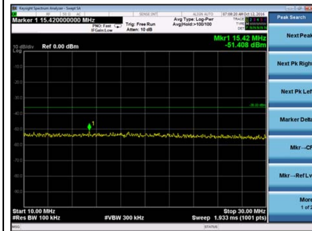
AIS1 10MHz - 30MHz
