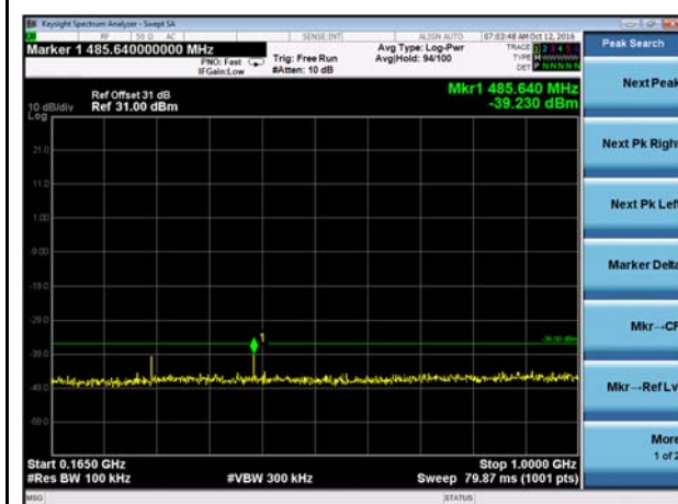
AIS1 165MHz - 1GHz
