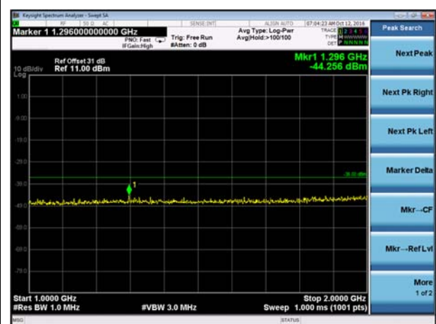
AIS1 1GHz - 2GHz
