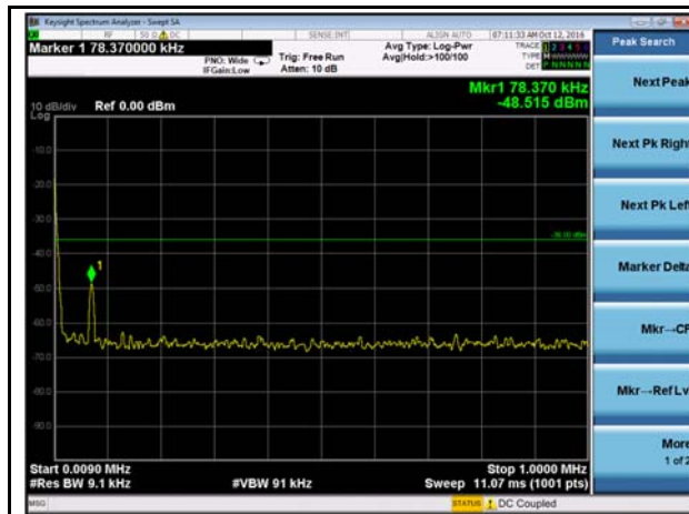
AIS2 9KHz - 1MHz
