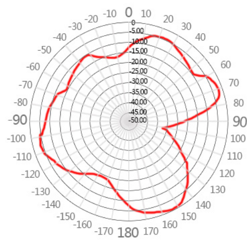
2400.000MHz
