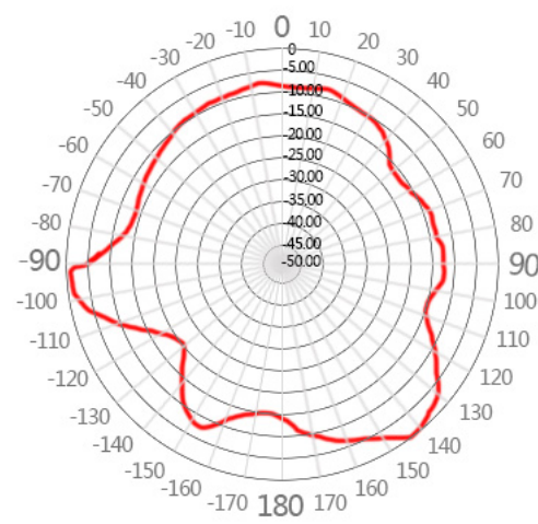
2450.000MHz
