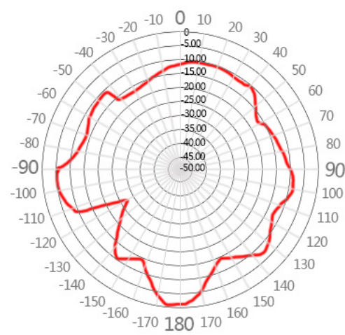
2500.000MHz
