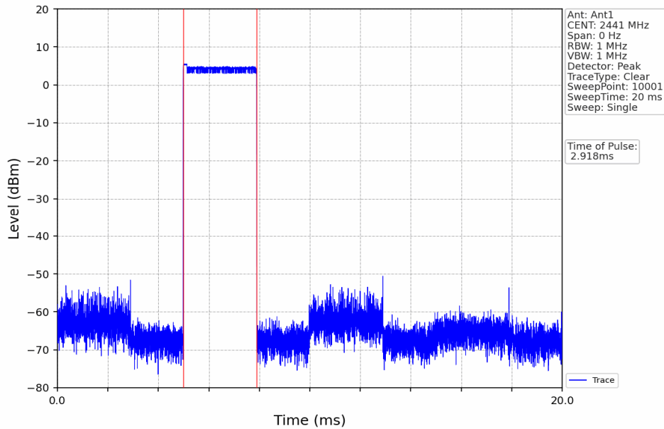
Pi/4DQPSK_2DH5_HOPP_Ant1_NTNV
