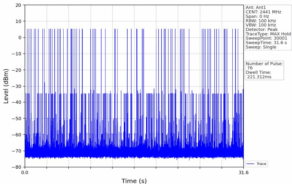
GFSK_DH5_HOPP_Ant1_NTNV
