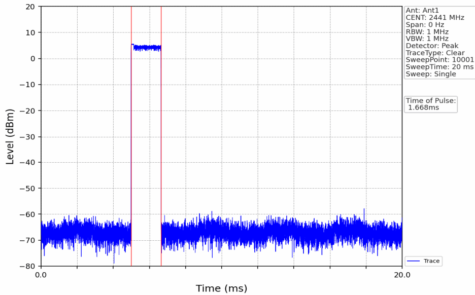
8DPSK_3DH3_HOPP_Ant1_NTNV
