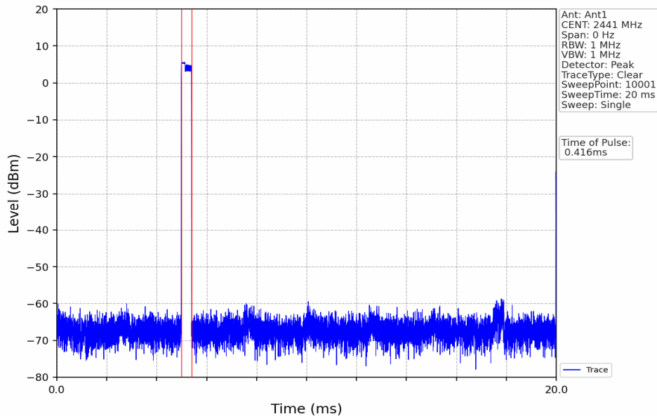
Pi/4DQPSK_2DH1_HOPP_Ant1_NTNV
