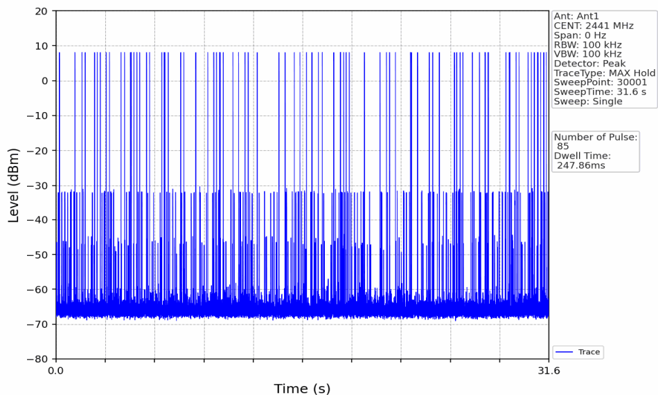
Pi/4DQPSK_2DH5_HOPP_Ant1_NTNV
