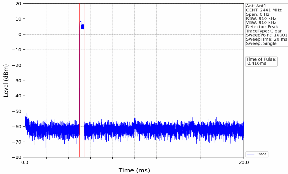
Pi/4DQPSK_2DH1_HOPP_Ant1_NTNV
