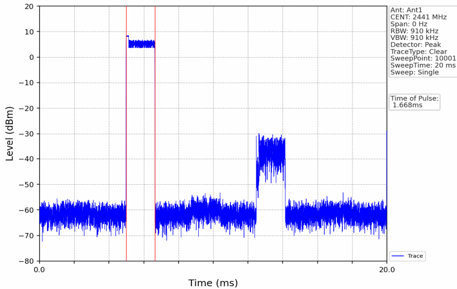
Pi/4DQPSK_2DH3_HOPP_Ant1_NTNV
