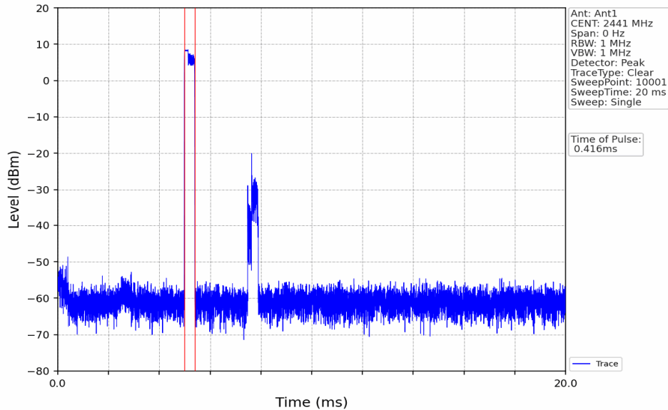
8DPSK_3DH1_HOPP_Ant1_NTNV
