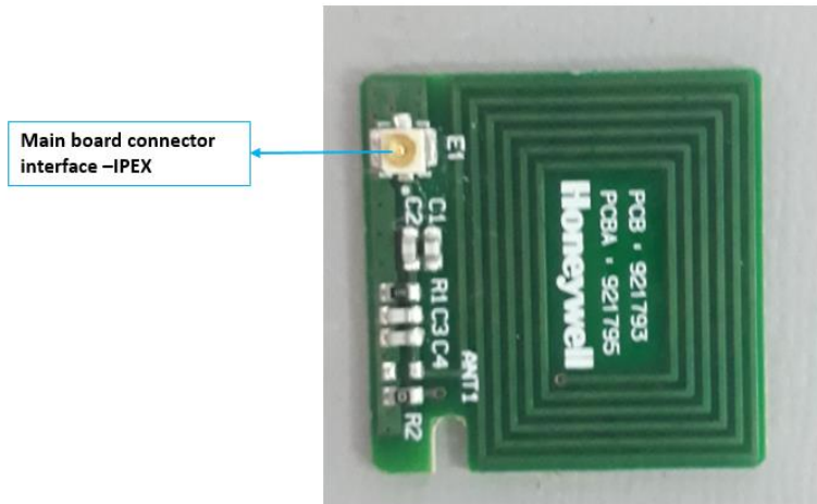
PCBA TOP SIDE
