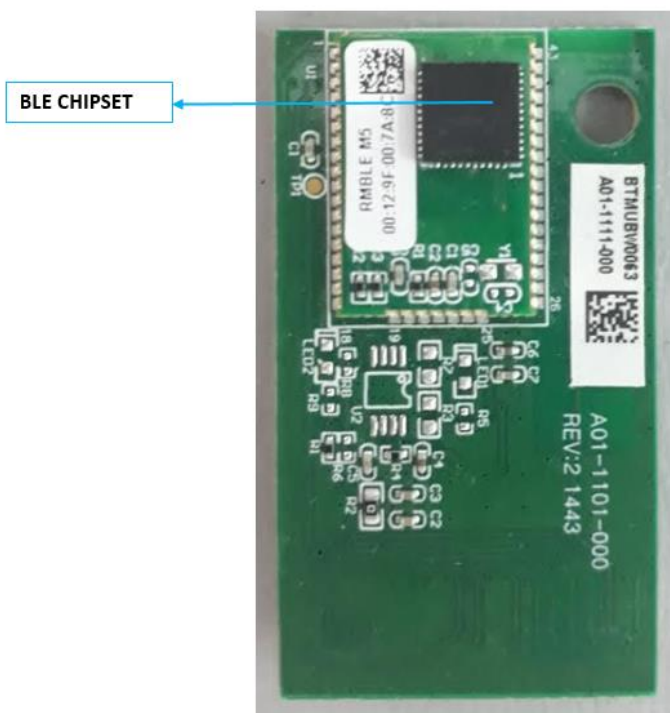
PCBA TOP SIDE
