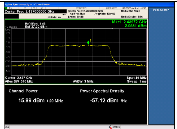
11n-20MHz-PWR-Mid-TX2
