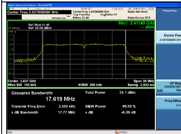
11n-20MHz-6dB BW-Mid
