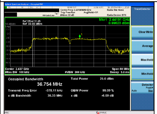
11n-40MHz-6dB BW-Mid
