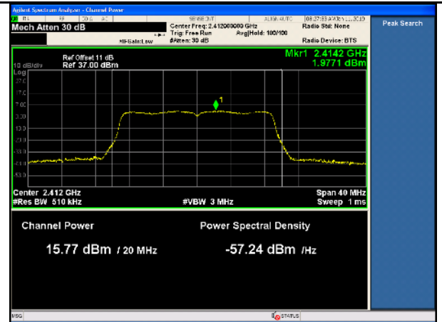
11n-20MHz-PWR-Low-TX2
