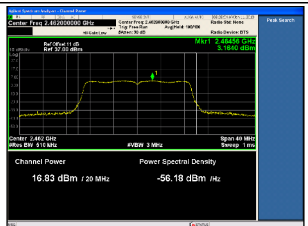
11n-20MHz-PWR-High-TX2
