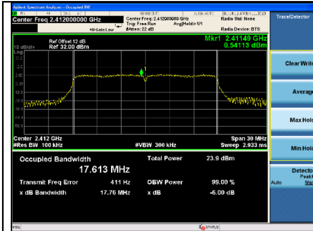
11n-20MHz-6dB BW-Low
