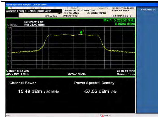
802.11a 5220MHz-PWR-TX1
