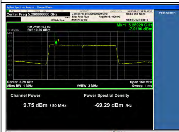
802.11ac-80MHz- 5290MHz-PWR-TX1
