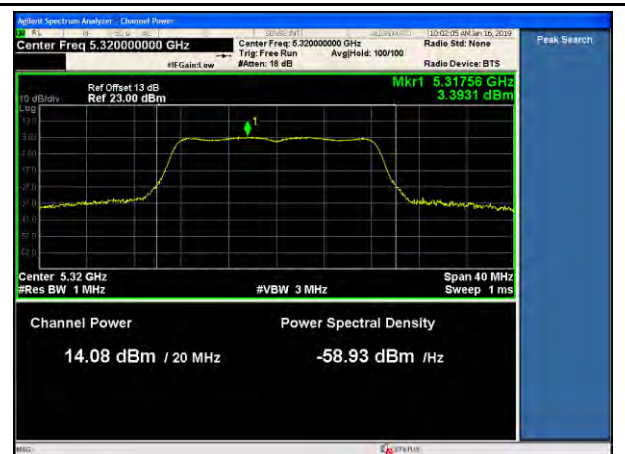
802.11a 5320MHz-PWR-TX2
