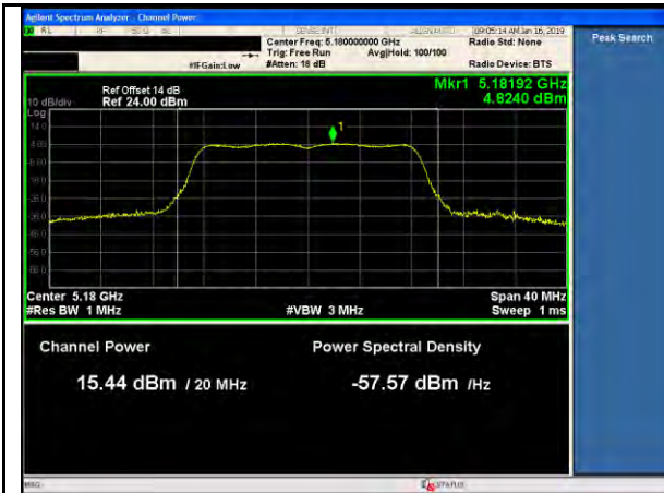
802.11a 5180MHz-PWR-TX1
