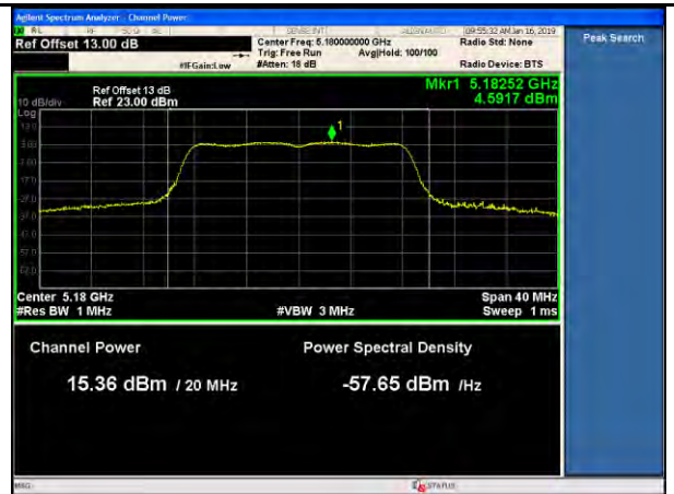
802.11a 5180MHz-PWR-TX2
