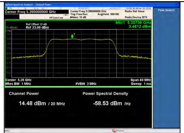
802.11a 5260MHz-PWR-TX2
