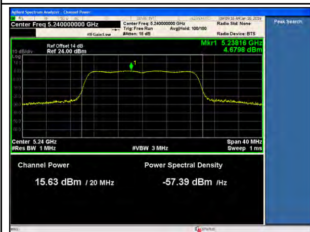
802.11n-20MHz- 5240MHz-PWR-TX1
