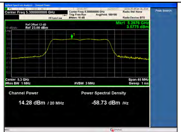
802.11a 5300MHz-PWR-TX2
