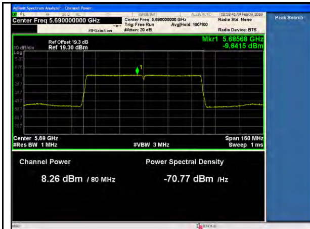
802.11ac-80MHz- 5690MHz-PWR-TX1
