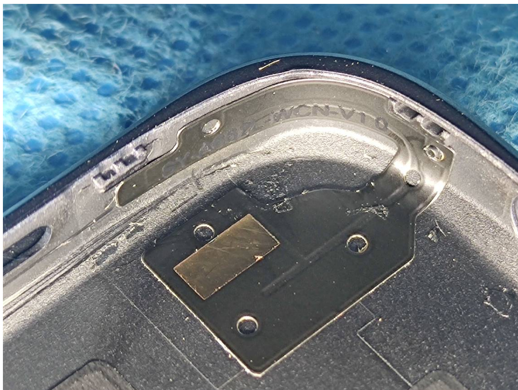
Bluetooth/WiFi Antenna
