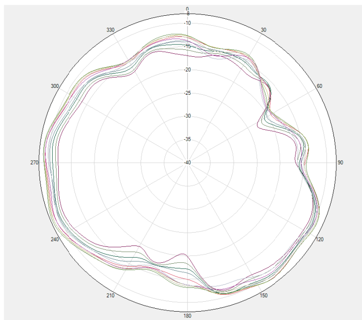
GSM850 / WCDMA B5 / LTE B5/B20/B26 \Phi=90\text{deg}
