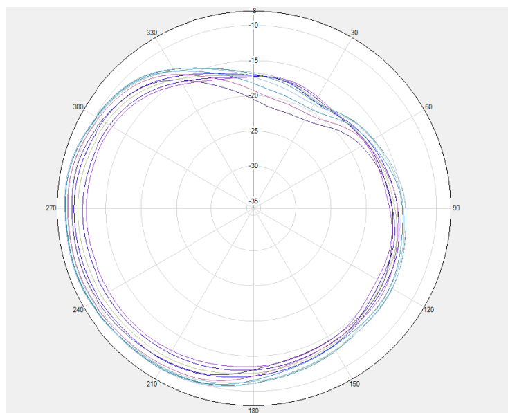
GSM850 / WCDMA B5 / LTE B5/B20/B26 \Theta=90\text{deg}
