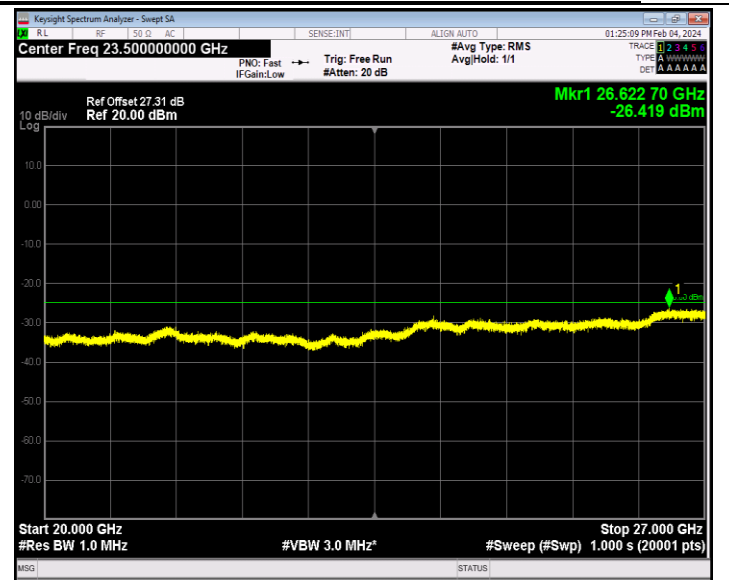
Band7_20MHz_QPSK_20850_1RB#0_20000~27000_20000~27000
