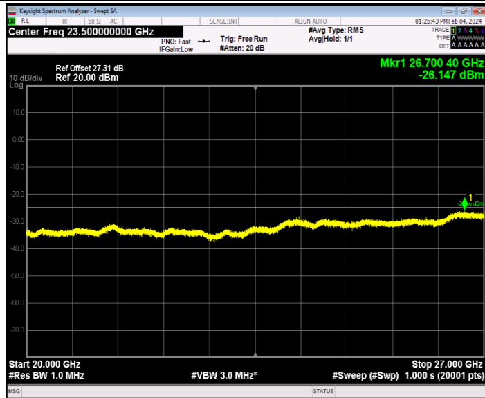
Band7_20MHz_16QAM_20850_1RB#0_20000~27000_20000~27 000
