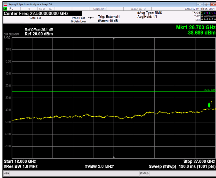
Band41_20MHz_16QAM_41140_1RB#0_18000~27000_18000~27000
