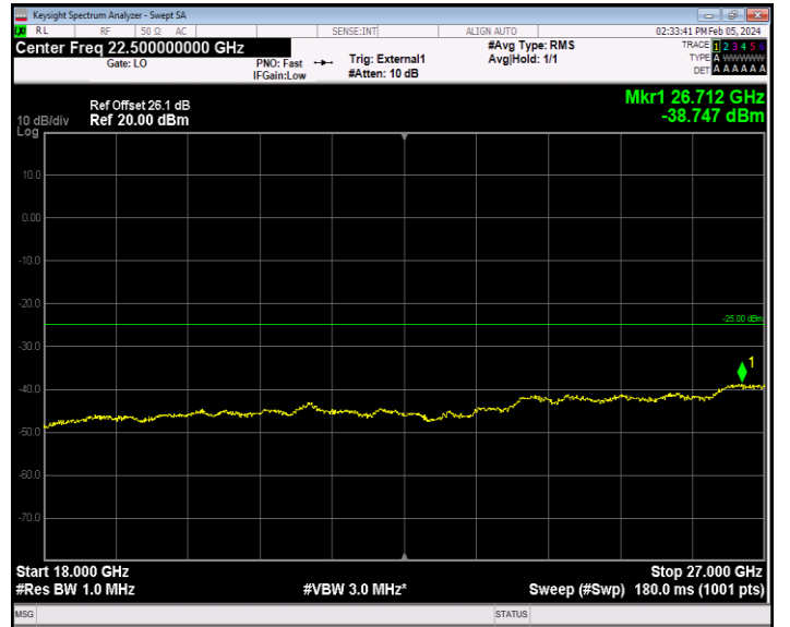
Band41_20MHz_64QAM_41140_1RB#0_18000~27000_18000~27000
