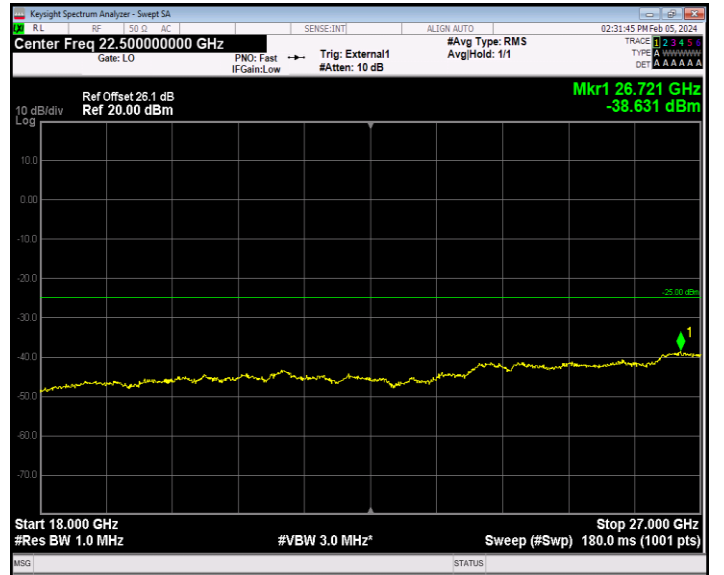
Band41_20MHz_16QAM_40640_1RB#0_18000~27000_18000~27000
