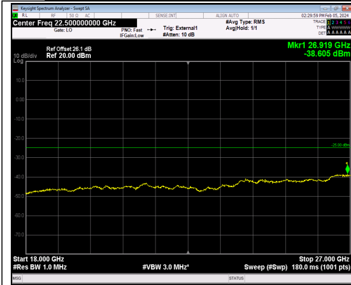
Band41_20MHz_16QAM_40140_1RB#0_18000~27000_18000~27000
