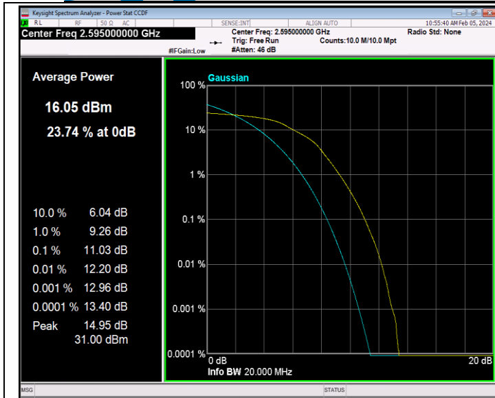
41(2535-2655)-20MHz-16QAM-40640-100RB#0-PASS
