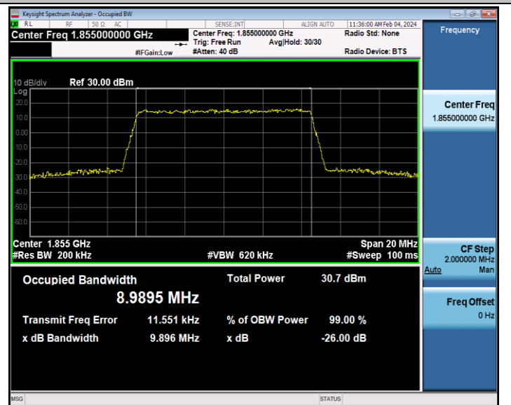
Band2-10MHz-QPSK-18650-50RB#0-PASS
