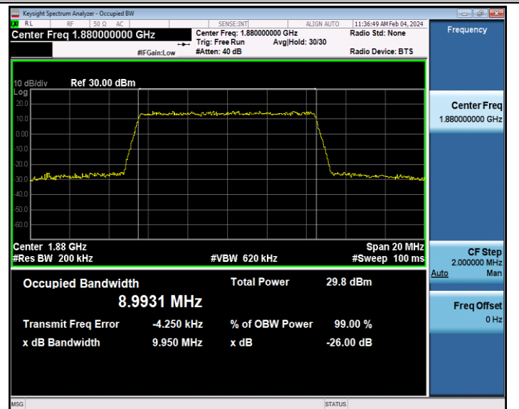
Band2-10MHz-16QAM-18900-50RB#0-PASS
