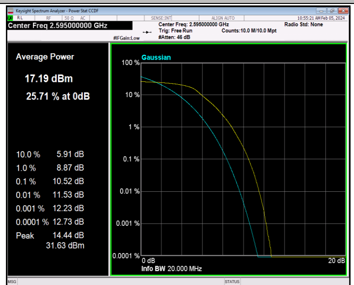
41(2535-2655)-20MHz-QPSK-40640-100RB#0-PASS
