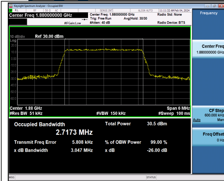
Band2-3MHz-QPSK-18900-15RB#0-PASS
