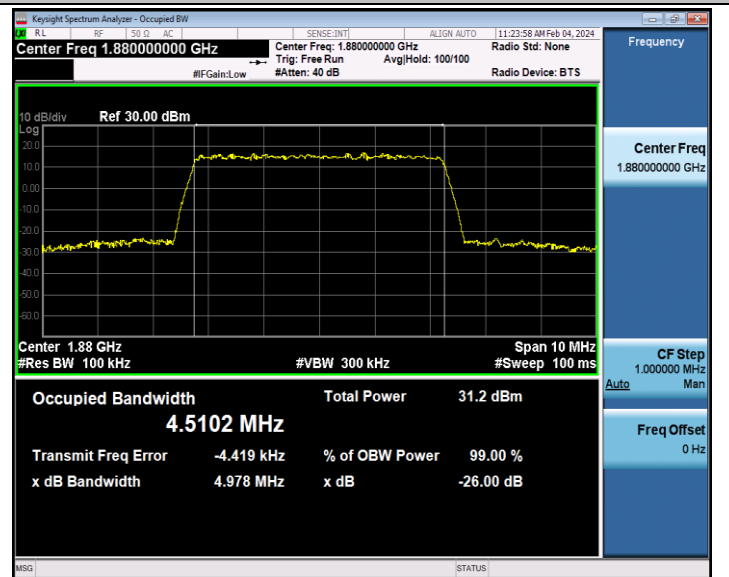
Band2-5MHz-QPSK-18900-25RB#0-PASS
