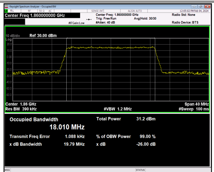
Band2-20MHz-QPSK-18700-100RB#0-PASS
