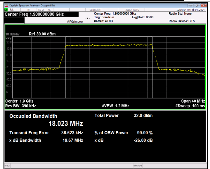
Band2-20MHz-QPSK-19100-100RB#0-PASS
