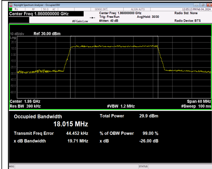
Band2-20MHz-16QAM-18700-100RB#0-PASS
