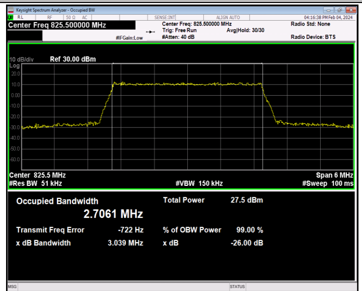
26(824-849)-3MHz-64QAM-26805-15RB#0-PASS
