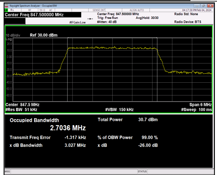
26(824-849)-3MHz-QPSK-27025-15RB#0-PASS
