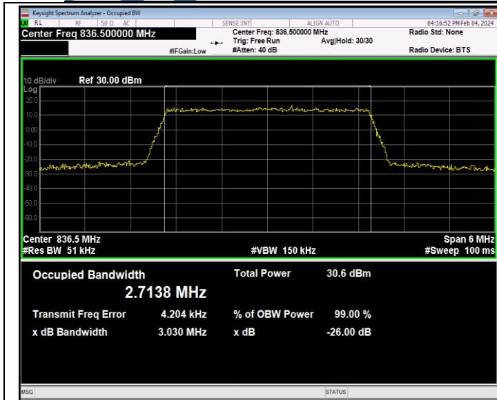
26(824-849)-3MHz-QPSK-26915-15RB#0-PASS
