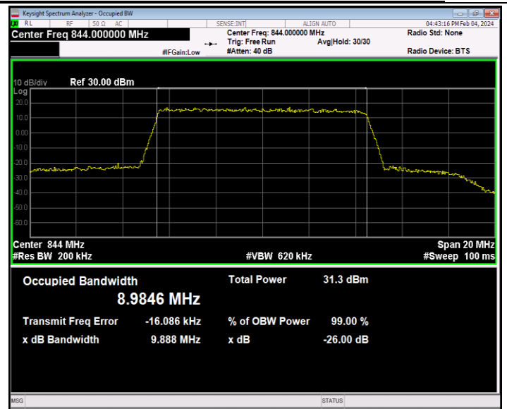
26(824-849)-10MHz-QPSK-26990-50RB#0-PASS
