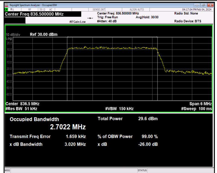
26(824-849)-3MHz-16QAM-26915-15RB#0-PASS
