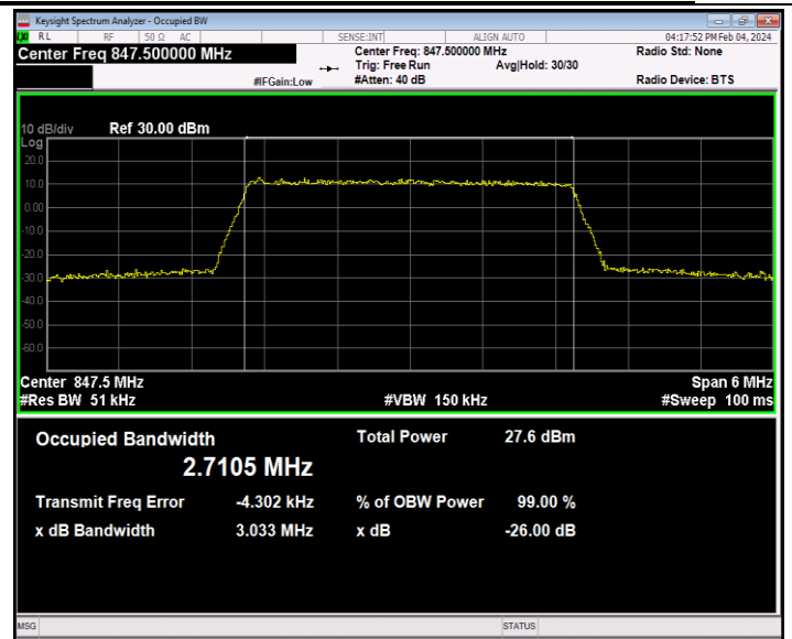
26(824-849)-3MHz-64QAM-27025-15RB#0-PASS
