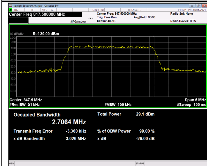
26(824-849)-3MHz-16QAM-27025-15RB#0-PASS
