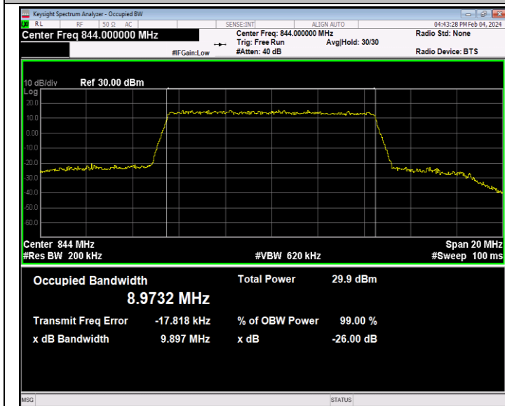
26(824-849)-10MHz-16QAM-26990-50RB#0-PASS
