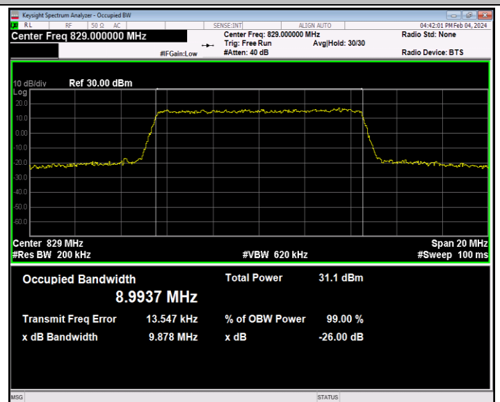
26(824-849)-10MHz-QPSK-26840-50RB#0-PASS
