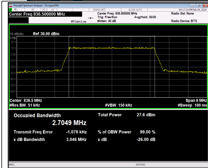
26(824-849)-3MHz-64QAM-26915-15RB#0-PASS
