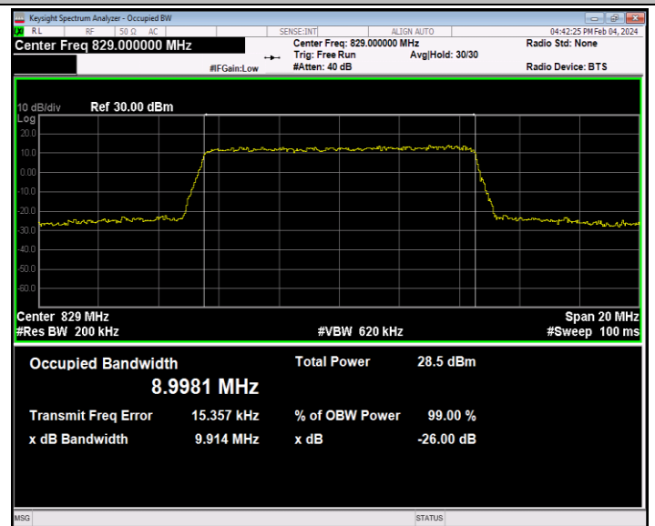
26(824-849)-10MHz-64QAM-26840-50RB#0-PASS
