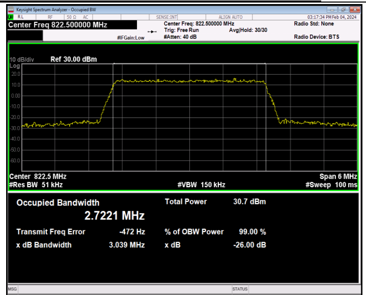
26(814-824)-3MHz-QPSK-26775-15RB#0-PASS
