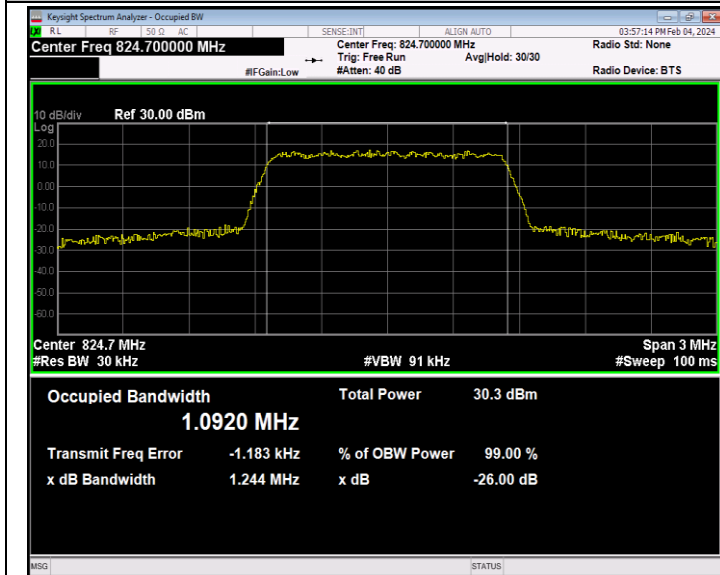
26(824-849)-1.4MHz-QPSK-26797-6RB#0-PASS
