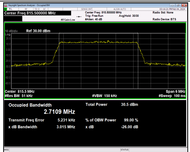
26(814-824)-3MHz-QPSK-26705-15RB#0-PASS
