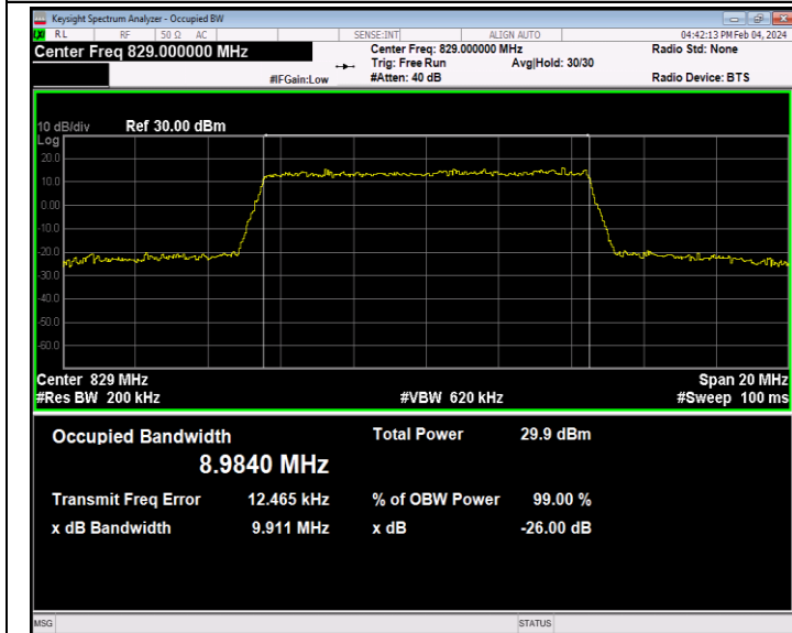
26(824-849)-10MHz-16QAM-26840-50RB#0-PASS
