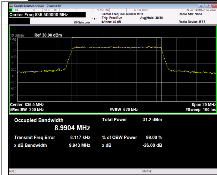
26(824-849)-10MHz-QPSK-26915-50RB#0-PASS
