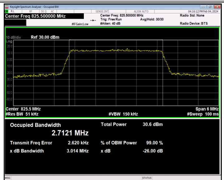
26(824-849)-3MHz-QPSK-26805-15RB#0-PASS
