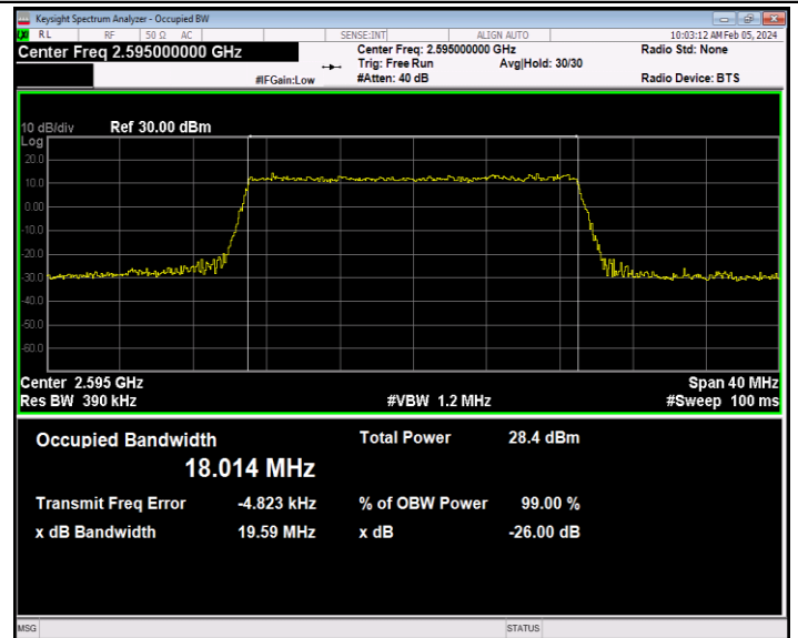
41(2535-2655)-20MHz-64QAM-40640-100RB#0-PASS
