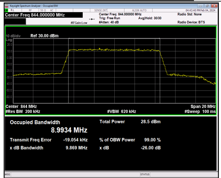
26(824-849)-10MHz-64QAM-26990-50RB#0-PASS
