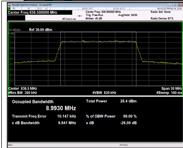
26(824-849)-10MHz-64QAM-26915-50RB#0-PASS
