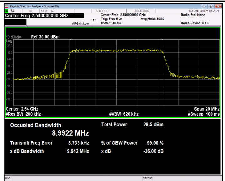
41(2535-2655)-10MHz-16QAM-40090-50RB#0-PASS
