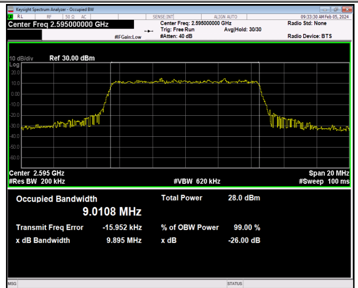
41(2535-2655)-10MHz-64QAM-40640-50RB#0-PASS
