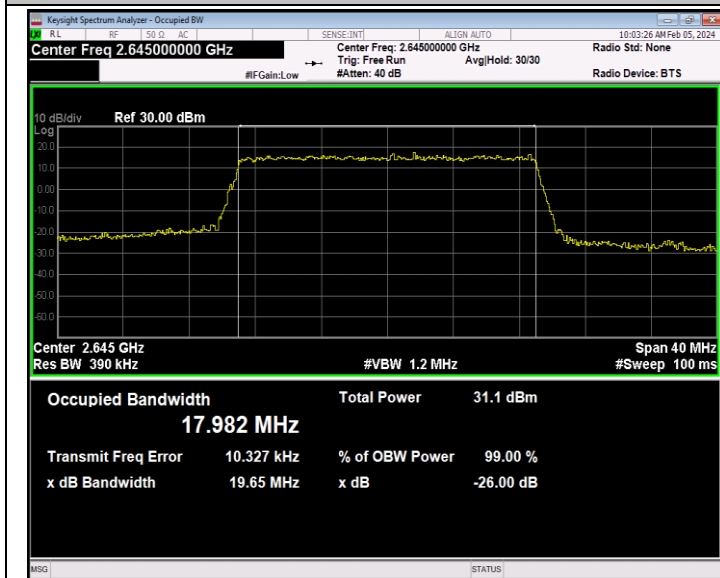
41(2535-2655)-20MHz-QPSK-41140-100RB#0-PASS
