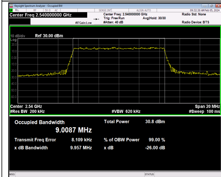
41(2535-2655)-10MHz-QPSK-40090-50RB#0-PASS
