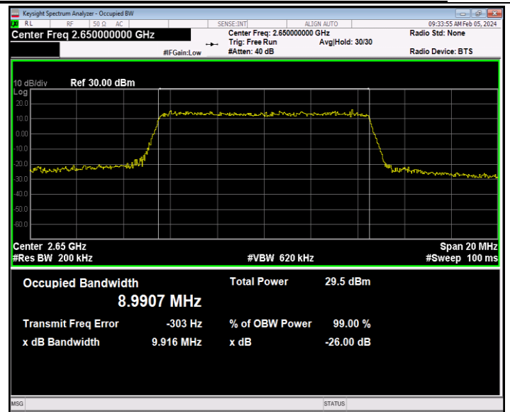
41(2535-2655)-10MHz-16QAM-41190-50RB#0-PASS
