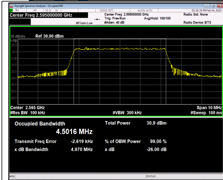
41(2535-2655)-5MHz-QPSK-40640-25RB#0-PASS
