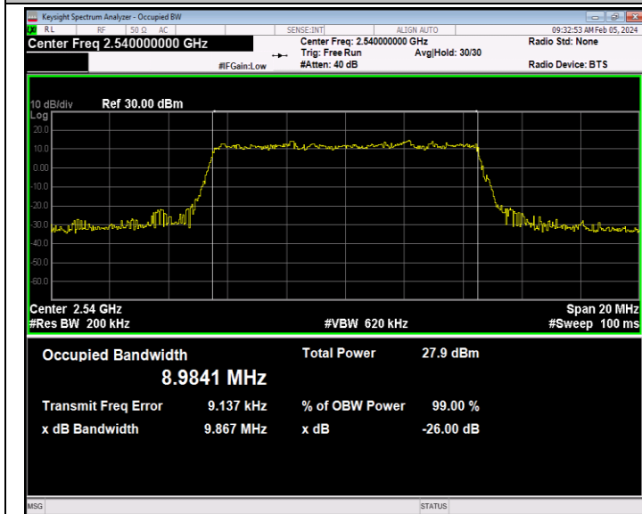
41(2535-2655)-10MHz-64QAM-40090-50RB#0-PASS
