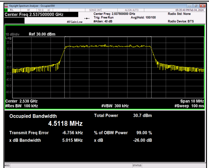
41(2535-2655)-5MHz-QPSK-40065-25RB#0-PASS
