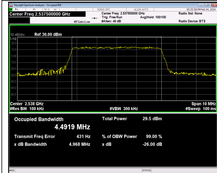
41(2535-2655)-5MHz-16QAM-40065-25RB#0-PASS
