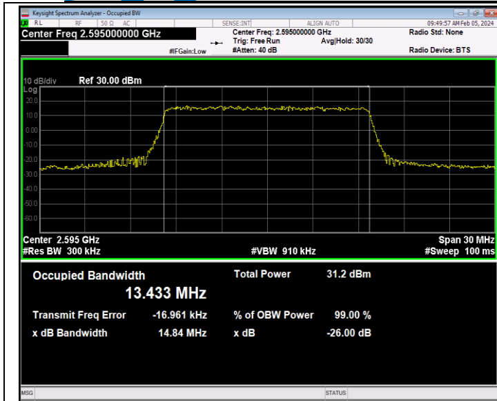
41(2535-2655)-15MHz-QPSK-40640-75RB#0-PASS
