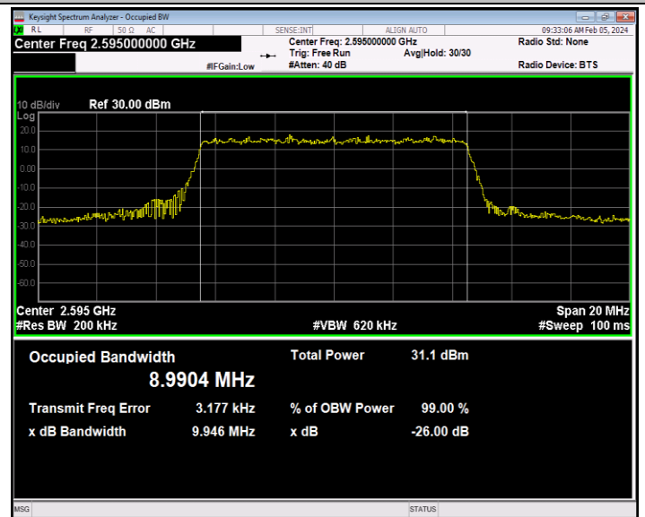
41(2535-2655)-10MHz-QPSK-40640-50RB#0-PASS
