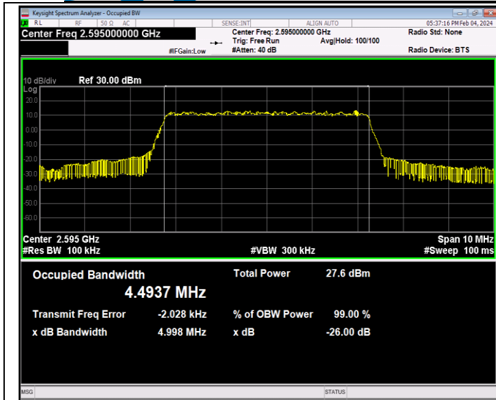
41(2535-2655)-5MHz-64QAM-40640-25RB#0-PASS
