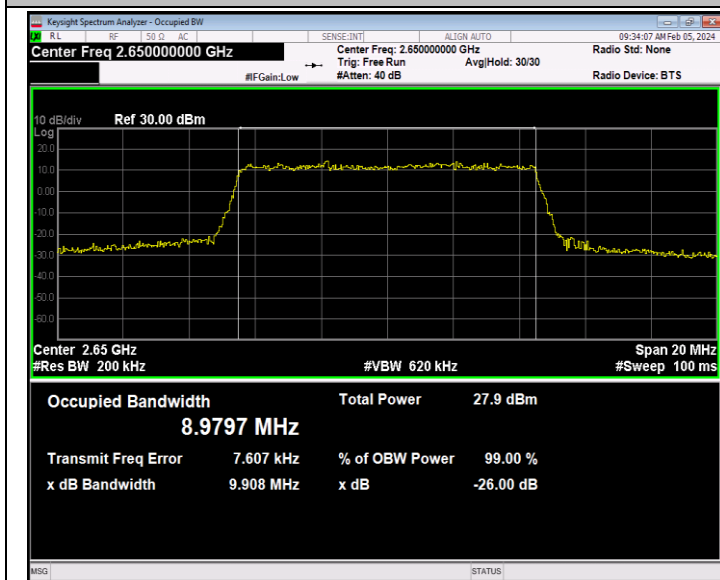
41(2535-2655)-10MHz-64QAM-41190-50RB#0-PASS
