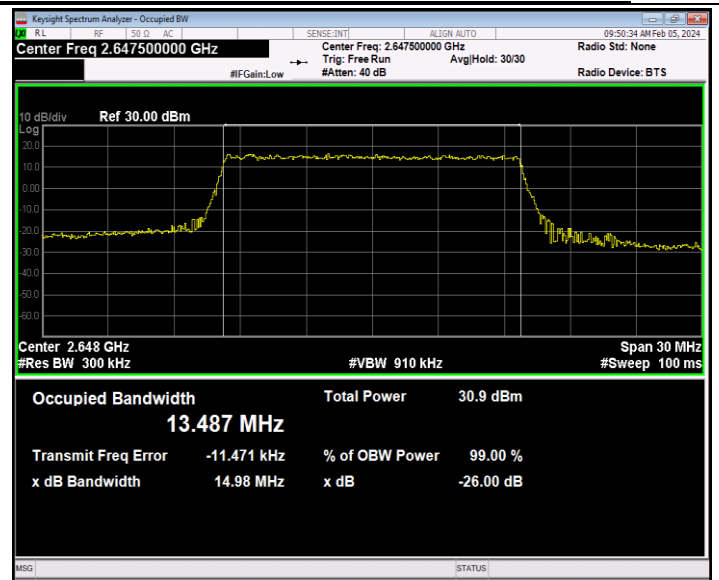
41(2535-2655)-15MHz-QPSK-41165-75RB#0-PASS
