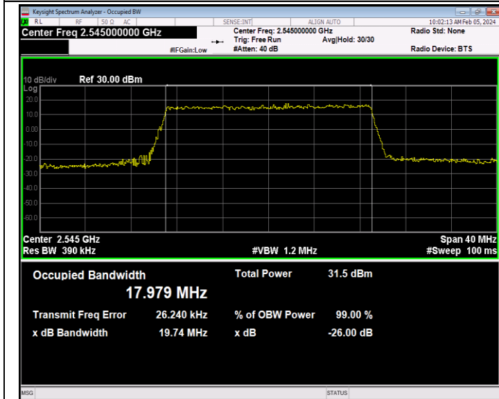
41(2535-2655)-20MHz-QPSK-40140-100RB#0-PASS
