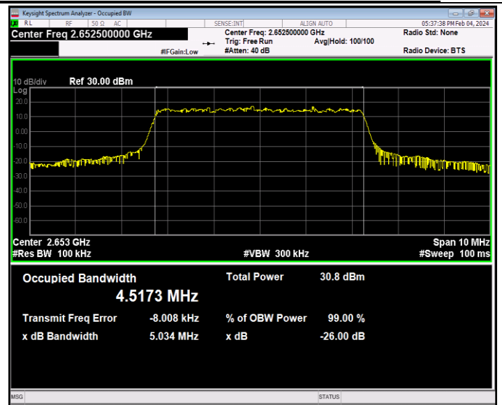
41(2535-2655)-5MHz-QPSK-41215-25RB#0-PASS
