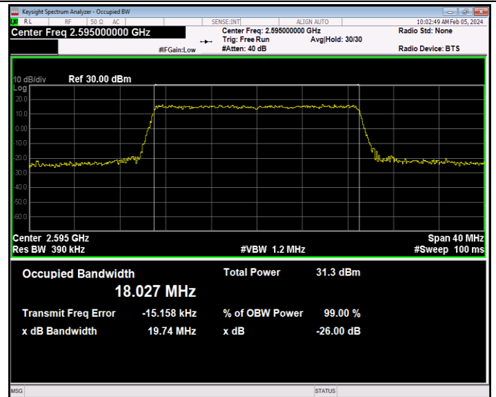
41(2535-2655)-20MHz-QPSK-40640-100RB#0-PASS
