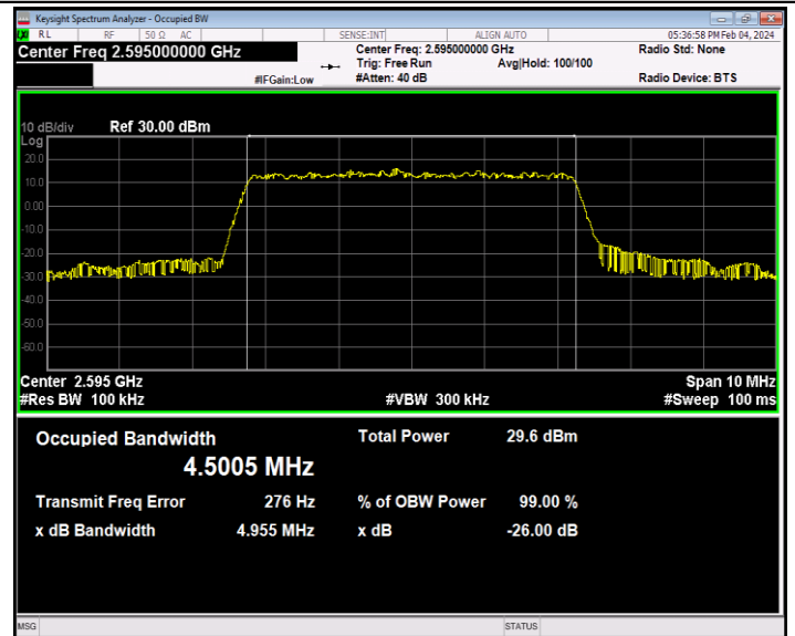
41(2535-2655)-5MHz-16QAM-40640-25RB#0-PASS
