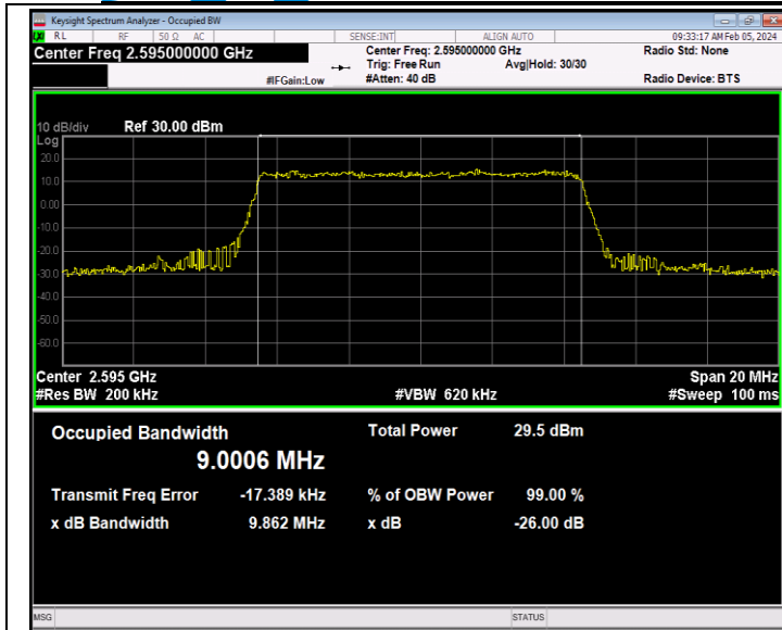
41(2535-2655)-10MHz-16QAM-40640-50RB#0-PASS
