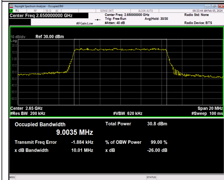
41(2535-2655)-10MHz-QPSK-41190-50RB#0-PASS
