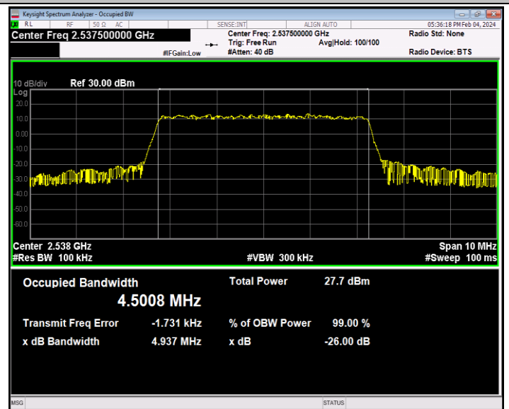
41(2535-2655)-5MHz-64QAM-40065-25RB#0-PASS
