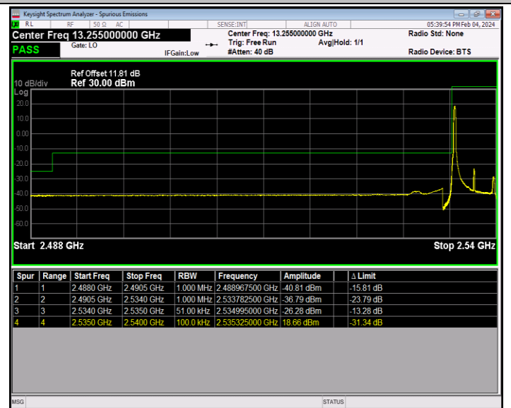
Band41_5MHz_QPSK_40065_1RB#0
