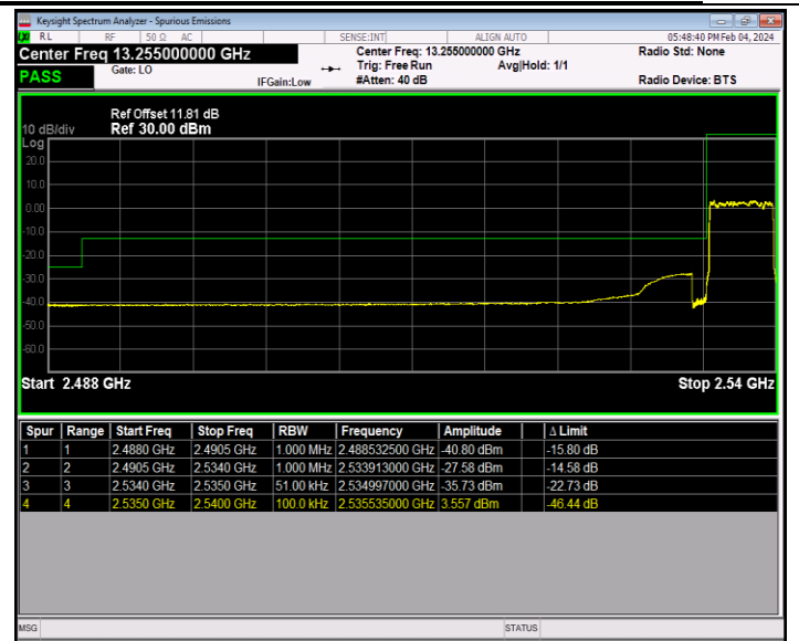
Band41_5MHz_QPSK_40065_25RB#0
