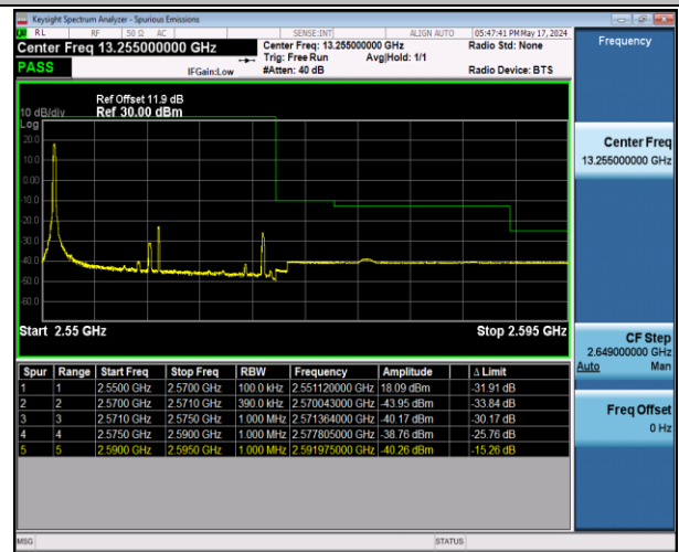
Band7_20MHz_16QAM_21350_1RB#0
