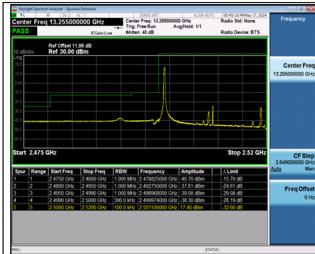
Band7_20MHz_16QAM_20850_1RB#0
