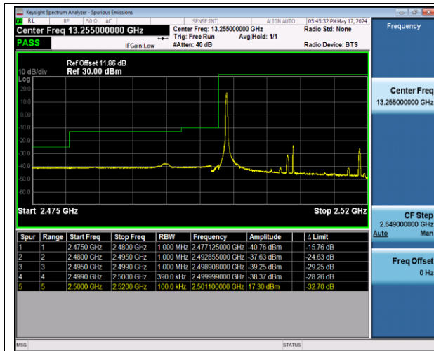
Band7_20MHz_64QAM_20850_1RB#0
