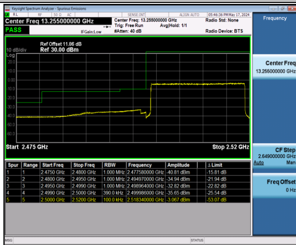
Band7_20MHz_QPSK_20850_100RB#0
