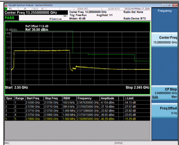
Band7_20MHz_16QAM_21350_100RB#0
