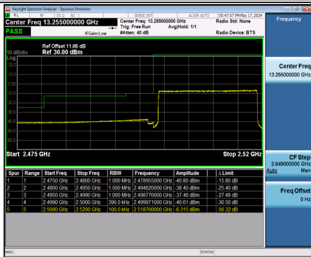
Band7_20MHz_64QAM_20850_100RB#0
