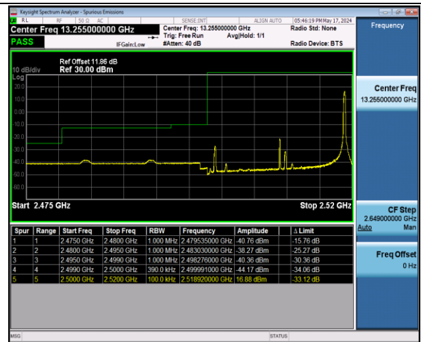
Band7_20MHz_64QAM_20850_1RB#99
