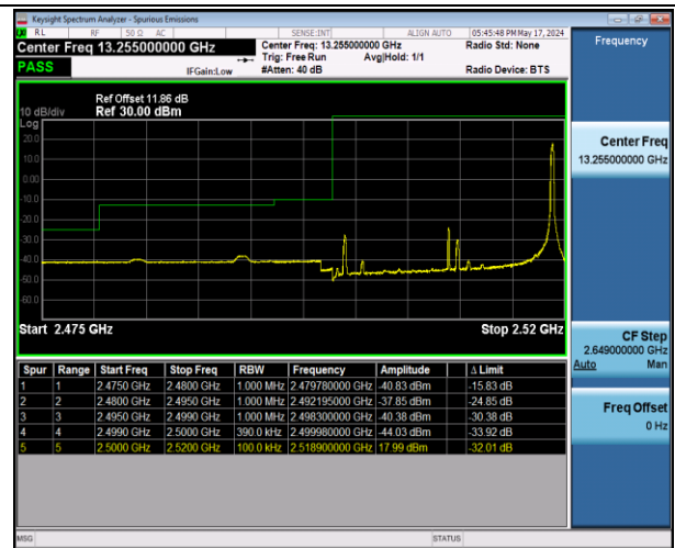
Band7_20MHz_QPSK_20850_1RB#99
