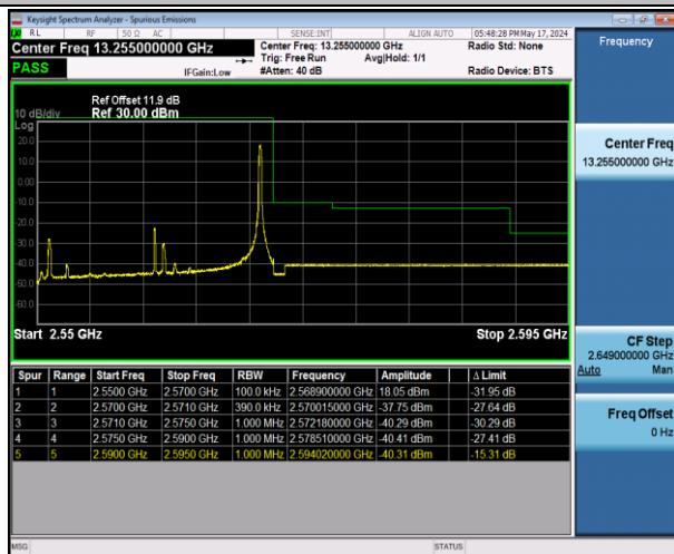
Band7_20MHz_16QAM_21350_1RB#99
