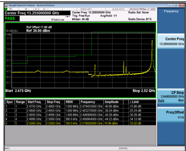
Band7_20MHz_16QAM_20850_1RB#99
