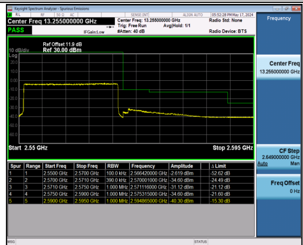
Band7_20MHz_QPSK_21350_100RB#0
