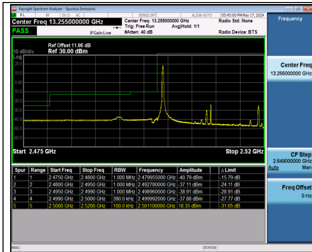
Band7_20MHz_QPSK_20850_1RB#0
