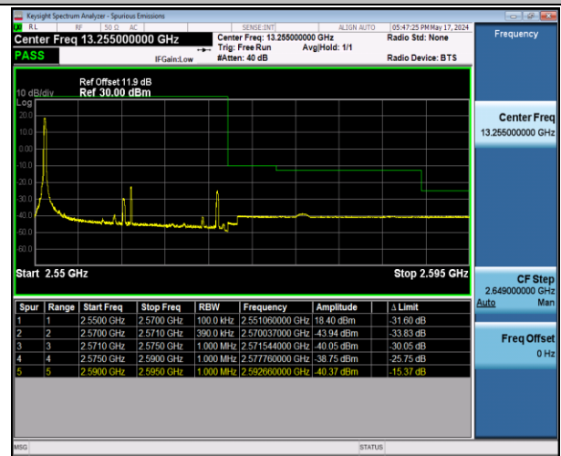
Band7_20MHz_QPSK_21350_1RB#0
