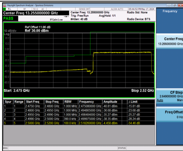
Band7_20MHz_16QAM_20850_100RB#0
