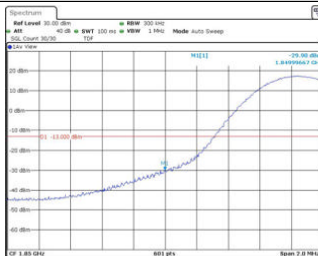
Band2-15MHz-16QAM-18675-1RB#74
