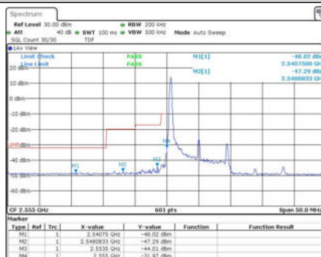
Band41-10MHz-QPSK-40290-1RB#0
