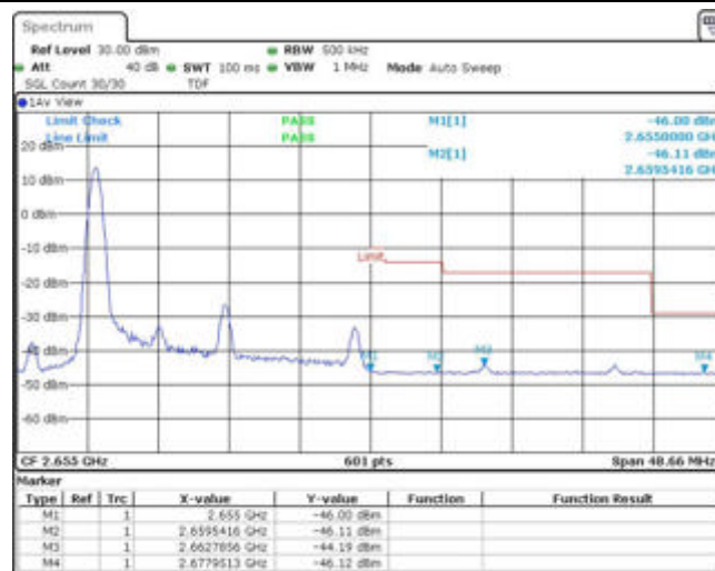
Band41-20MHz-QPSK-41140-1RB#99
