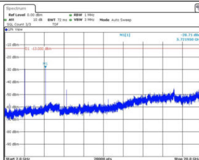
Band2-3MHz-QPSK-19185-1RB#0-Range3:2000~20000MHz
