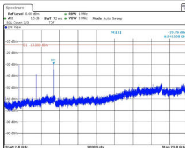
Band4-3MHz-QPSK-19965-1RB#0-Range3:2000~20000MHz
