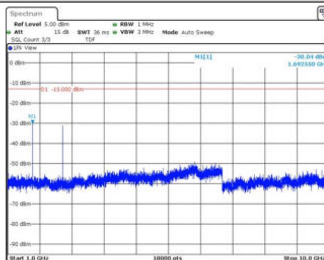
Band5-3MHz-QPSK-20635-1RB#0-Range2:1000~10000MHz
