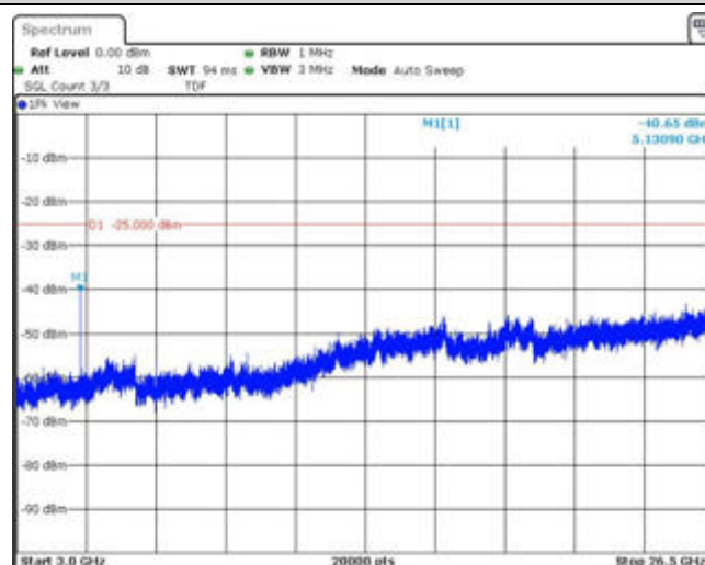
Band7-5MHz-QPSK-21425-1RB#0-Range3:3000~26500MHz
