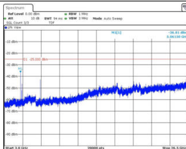
Band7-10MHz-QPSK-21100-1RB#0-Range3:3000~26500MHz
