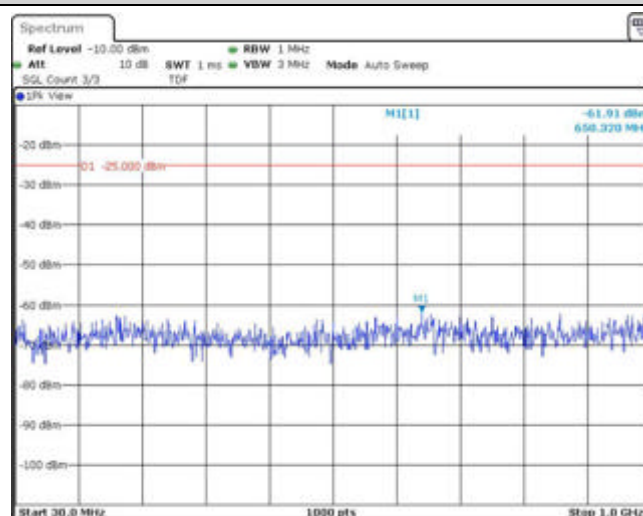
Band7-5MHz-QPSK-20775-1RB#0-Range2:1000~3000MHz
