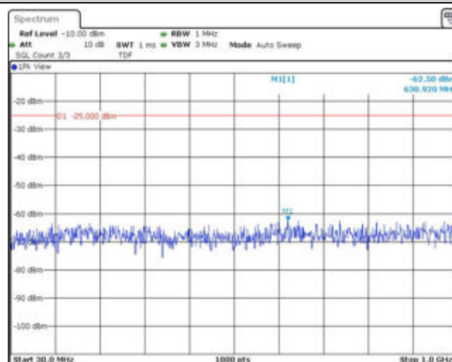
Band41-10MHz-QPSK-40290-1RB#0-Range1:30~1000MHz
