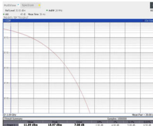
Band41-20MHz-QPSK-40590-100RB#0
