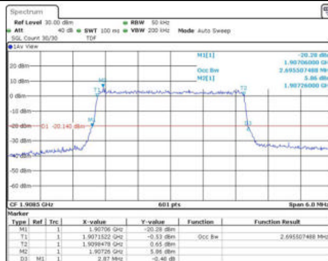
Band2-3MHz-16QAM-18615-15RB#0
