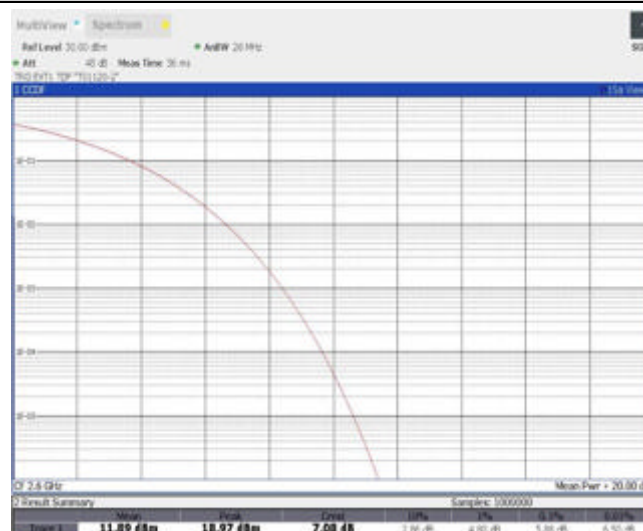
Band41-20MHz-QPSK-41140-1RB#0
