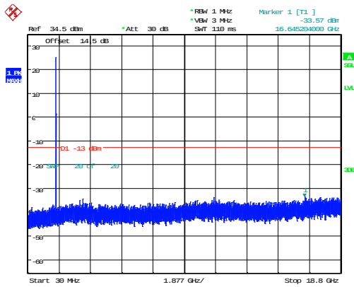
5MHz_Low_QPSK_1@0(30MHz~18.8GHz)
