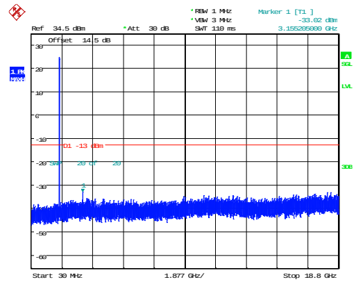
5MHz_Middle_QPSK_1@0(30MHz~18.8GHz)
