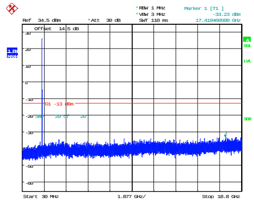
10MHz_Low_QPSK_1@0(30MHz~18.8GHz)
