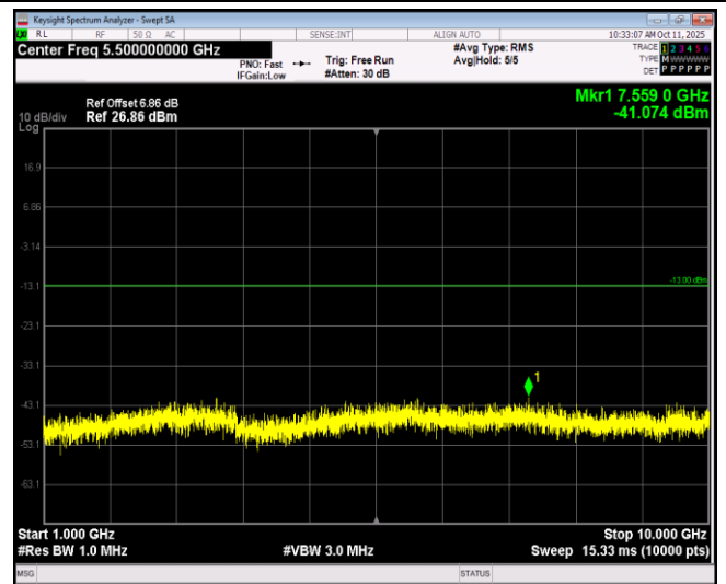
Band26-1.4MHz-QPSK-26697-1RB#0-Range2:1000~10000MHz
