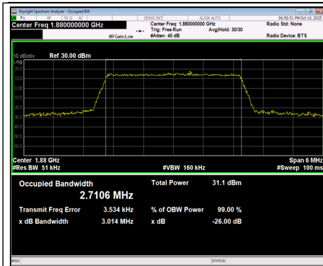
Band2-3MHz-16QAM-18615-15RB#0
