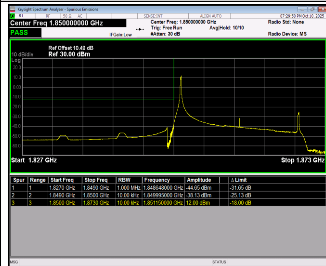
Band2-20MHz-QPSK-18700-100RB#0
