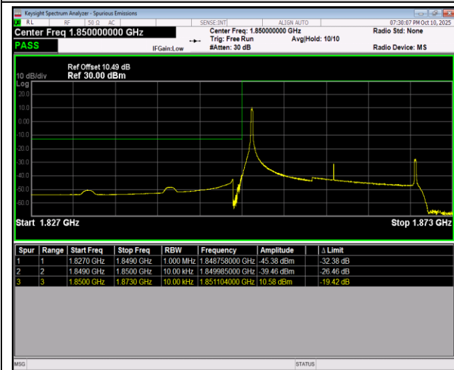
Band2-20MHz-16QAM-18700-100RB#0
